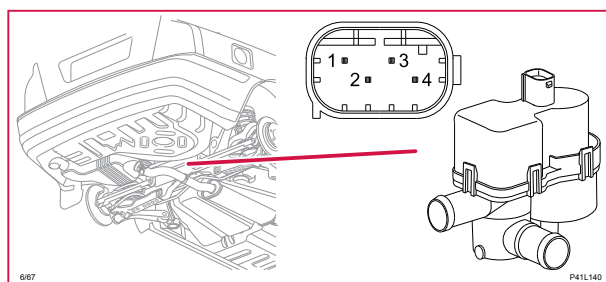
6/67 Pump bränsleläckagekontroll
