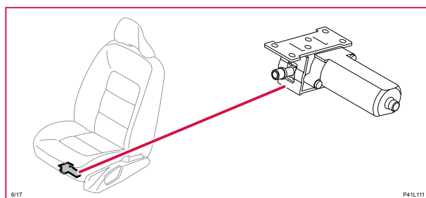
6/17 Sätesslutningsmotor, förarsida
