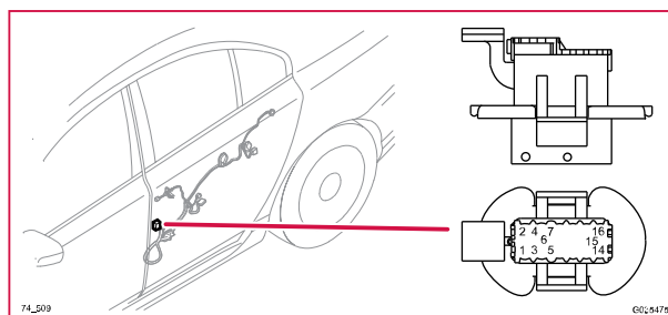
74/509 Kontaktstycke, BK
