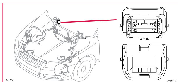
74/504 Kontaktstycke, WH
