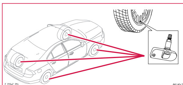
7/210-213 Däcktrycksgivare
