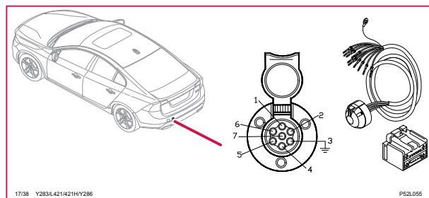
17/38 Uttag 7-poligt, ledningsmatta dragkrok
