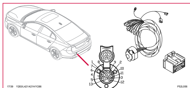
17/39 Uttag 13-poligt, ledningsmatta dragkrok
