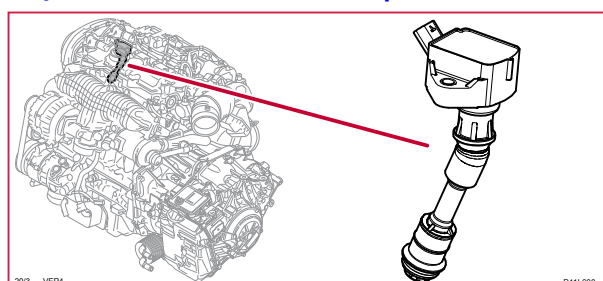
20/3-7 Tändstift med tändspolar
