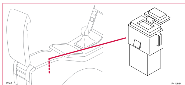
17/42 USB-port, tillbehör
