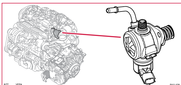
8/77 Reglerventil bränslevolym
