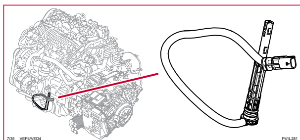
7/35 Givare oljenivå
