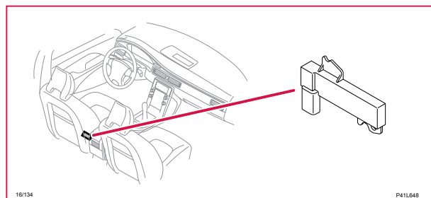
16/134 Antenn dörrlås kupé 2
