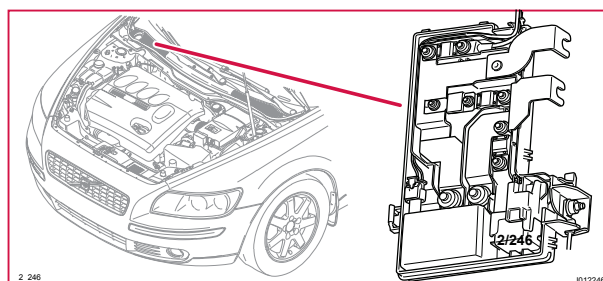
2/246 Relä, sekundärbatteri
