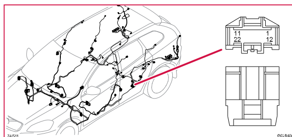
74/511 Kontaktstycke, GY
