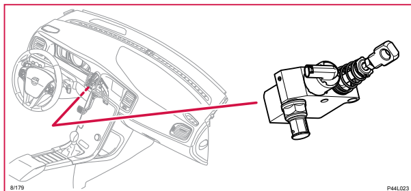
8/179 Bromspedalavstängningsventil
