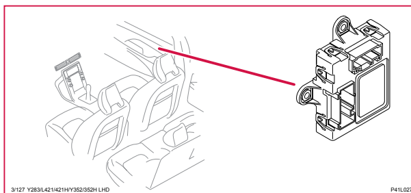
3/127 Styrenhet passagerardörr (PDM), LHD
