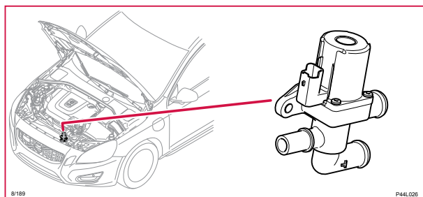
8/189 Ventil batterikylning 1
