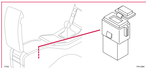
17/42 USB-port, tillbehör
