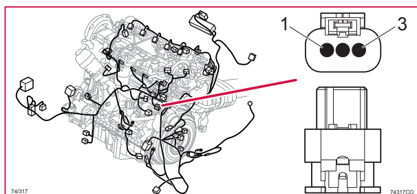
74/317 Kontaktstycke, BK
