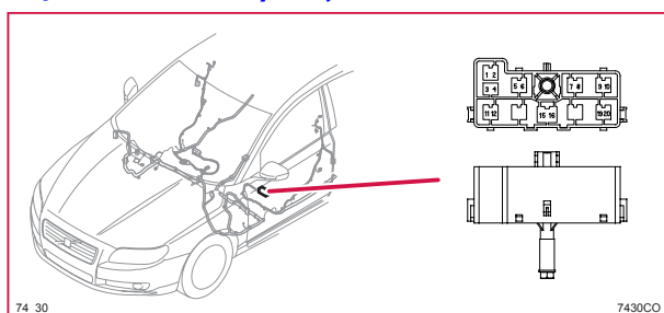
74/30 Kontaktstycke, BK
