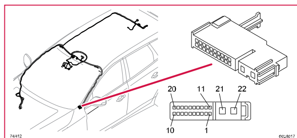
74/412 Kontaktstycke, GY
