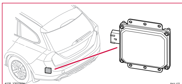
4/126 Styrenhet hinderdetektering vänster (SODL), V60H
