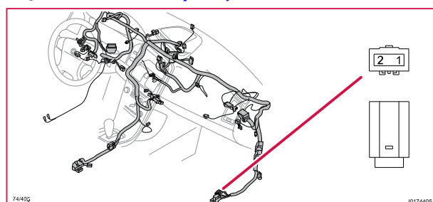
74/405 Kontaktstycke, WH
