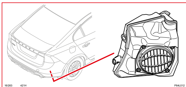
16/263 Bakre högtalare exteriört ljud
