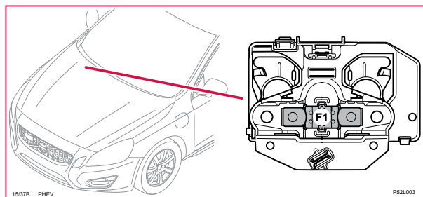
15/37B Elcentral motorrum
