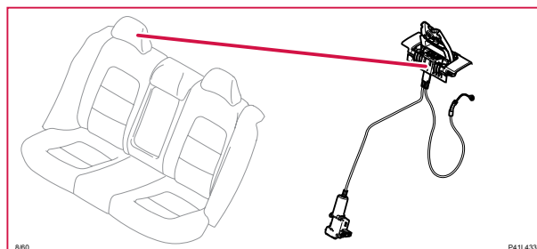
8/60 Solenoid nackstöd, bakre höger
