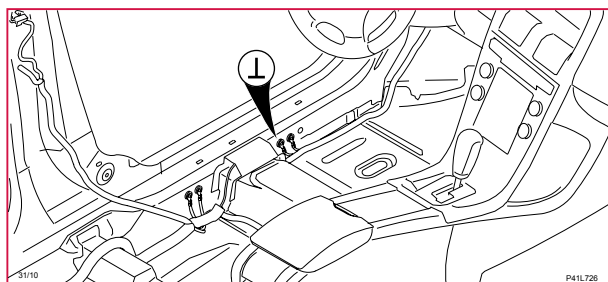
31/10 Stomanslutning, A-stolpe passagerarsida
