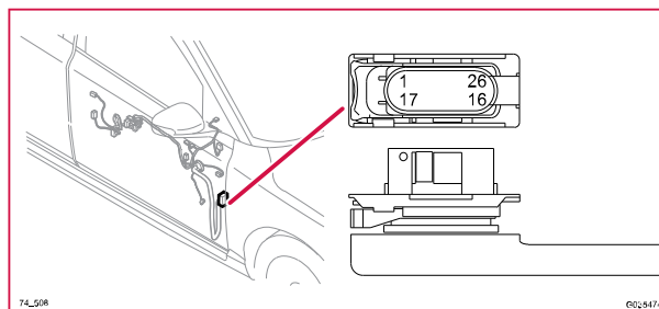
74/508 Kontaktstycke, BK
