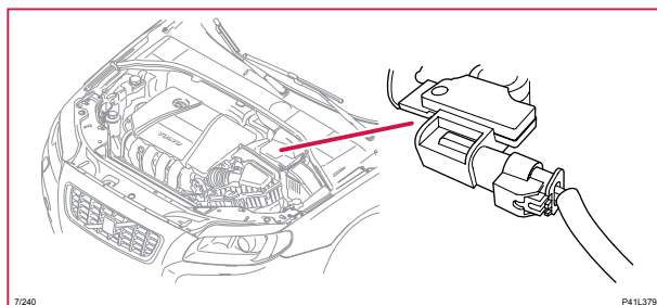
7/240 Batteriövervakningssensor (BMS)
