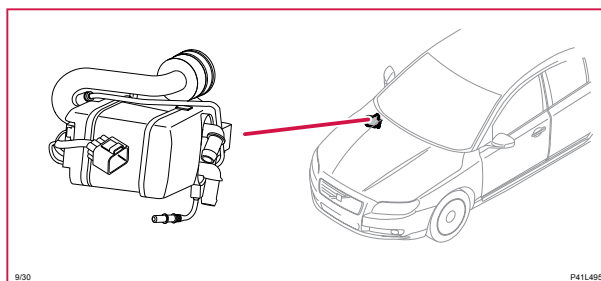
9/30 Tillskottsvärmare
