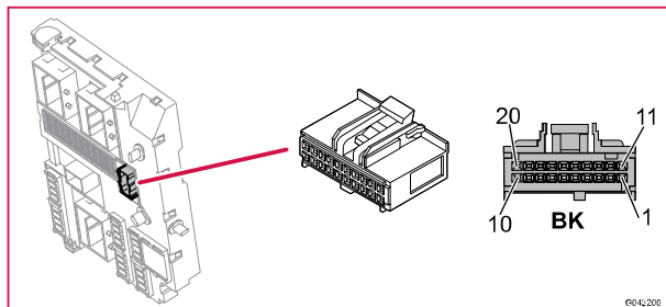
4/56:C4 Central elektronikstyrenhet (CEM)
