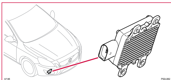
4/146 Styrenhet växellådaoljepump
