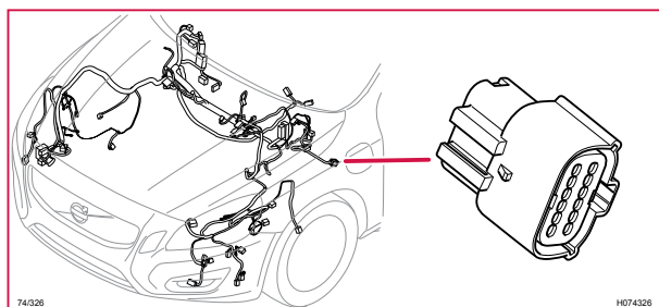
74/326 Kontaktstycke, BK
