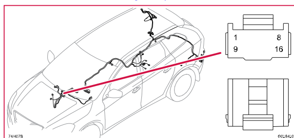
74/407B Kontaktstycke, GN
