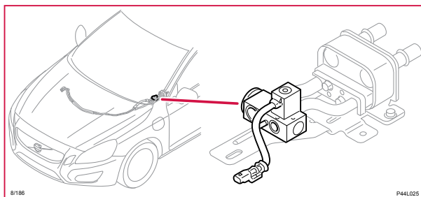
8/186 Avstängningsventil kylmedium
