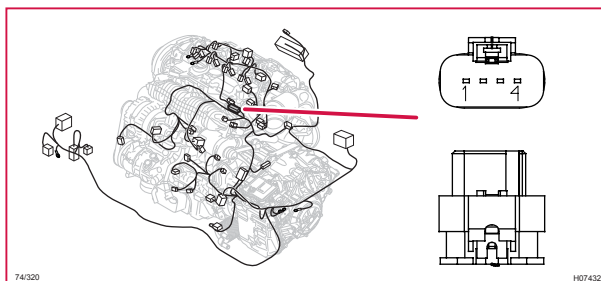
74/320 Kontaktstycke, BK, S60LH
