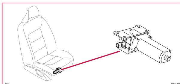
6/21 Säteslutningsmotor, passagerarsida
