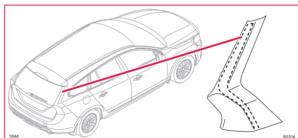
10/44 Bakljuslampa 1, höger
