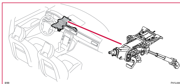
8/99 Tändare styrkolonn
