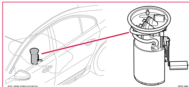
6/33 Bränslepump, S60LH
