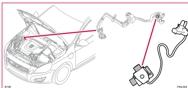
8/185 Klimatavstängningsventil
