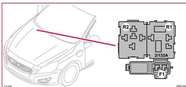
2/133A Relä A vakuumpump
