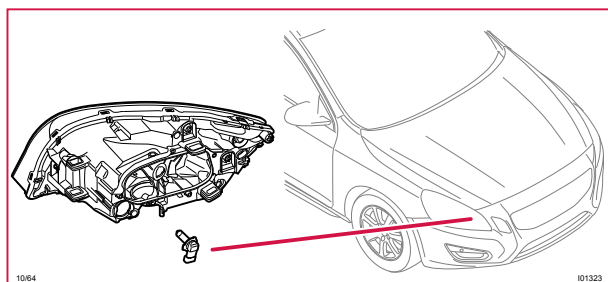
10/64 Helljus höger
