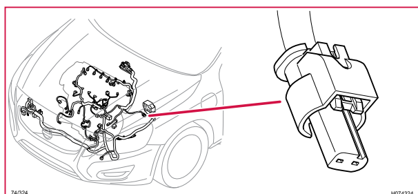
74/324 Kontaktstycke, BK, V60H
