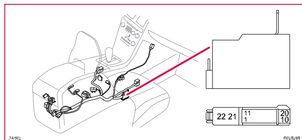
74/503 Kontaktstycke, GY, FOUR-C
