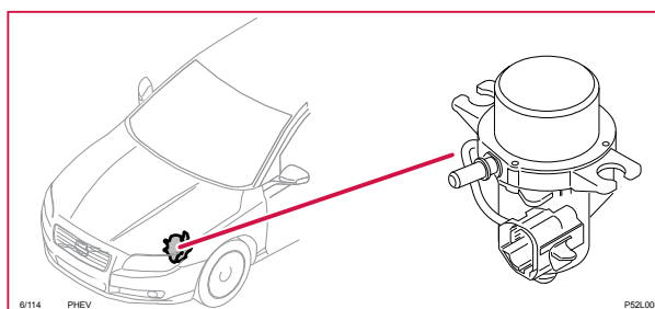
6/114 Vakuumpump
