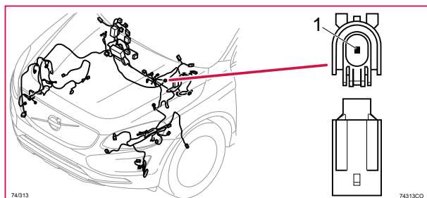
74/313 Kontaktstycke, BK, BMS
