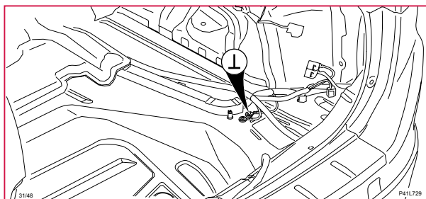
31/48 Stomanslutning, bakstam höger
