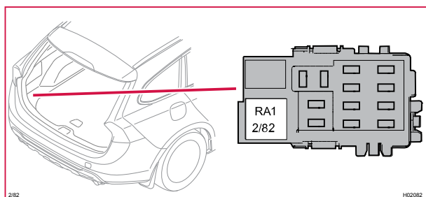
2/82 Relä eluppvärmd bakruta
