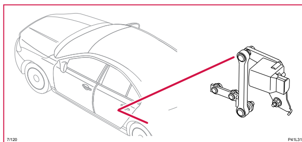
7/120 Höjdgivare hjulupphängning bak vänster
