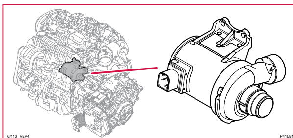
6/113 Kylvattenpump, S60LH
