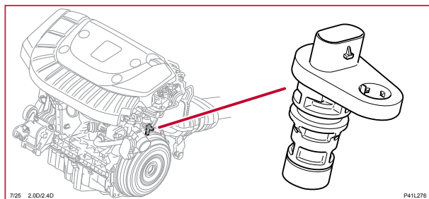
7/25 Impulsgivare, V60H
