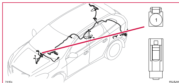
74/406 Kontaktstycke, VT
