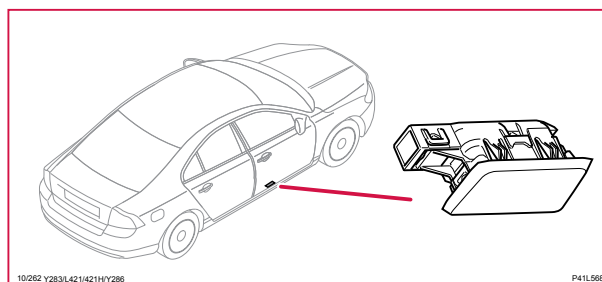
10/262 Markbelysning, passagerarsida, S60LH
