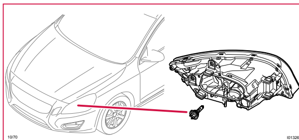
10/70 Halvljus vänster
