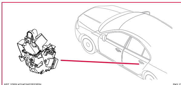
6/57 Motor, centrallås, bakdörr vänster
