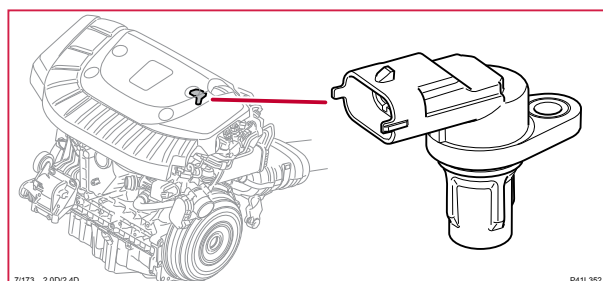
7/173 Lägesgivare kamaxel utloppssida, V60H
