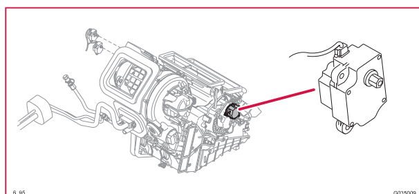
6/95 Styrenhet spjällmotor (DMM), temperatur vänster sida
