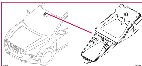
4/125 Styrenhet kollisionshastighet (CVM)
