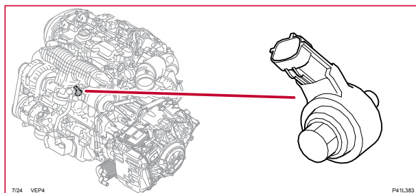
7/24 Knackgivare främre, S60LH
