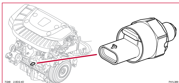
7/248 Oljetryck och temperaturgivare, V60H
