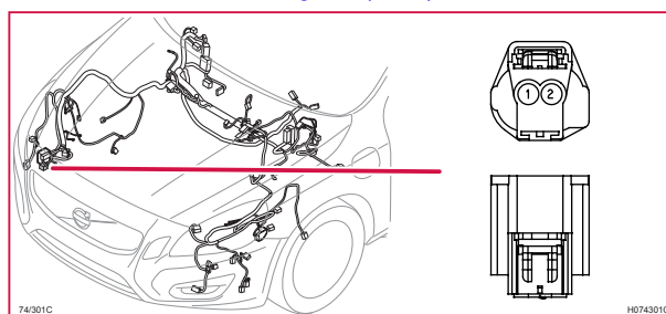
74/301C Kontaktstycke, GY, V60H
