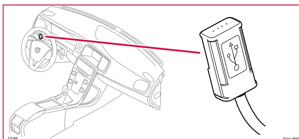
17/46 USB-port, Infotainment mjukvarunedladdning
