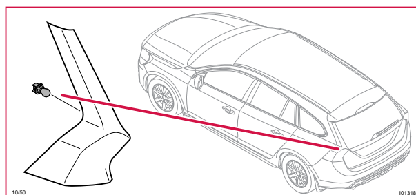
10/50 Bromsljus vänster
