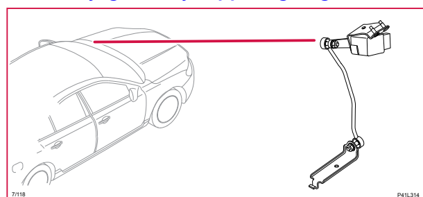
7/118 Höjdgivare hjulupphängning fram vänster
