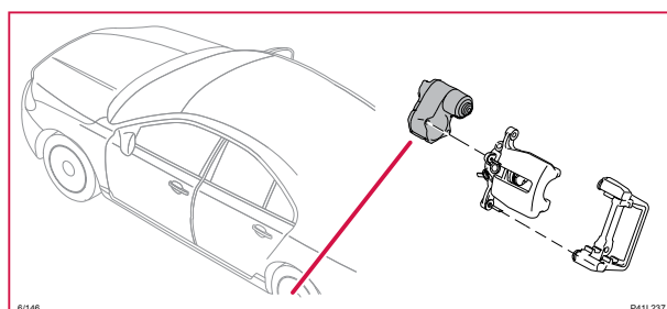
6/146 Elmotor bromsok, parkeringsbroms, bakre vänster
