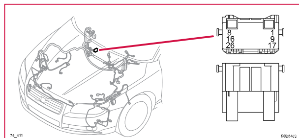
74/411 Kontaktstycke, GY
