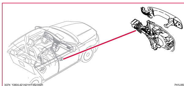
3/274 Låskontakt, höger framdörr
