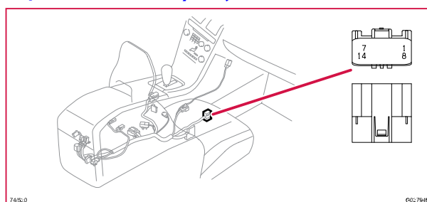
74/530 Kontaktstycke, GY
