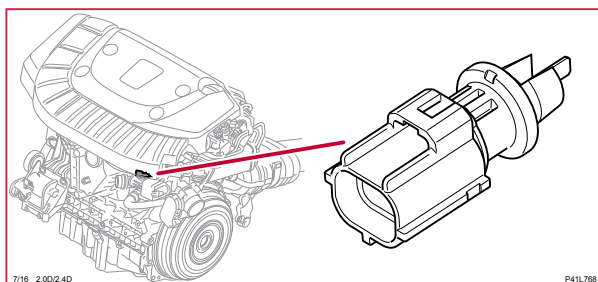
7/16 Givare kylvätsketemperatur, V60H
