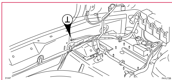
31/47 Stomanslutning, bakstam vänster
