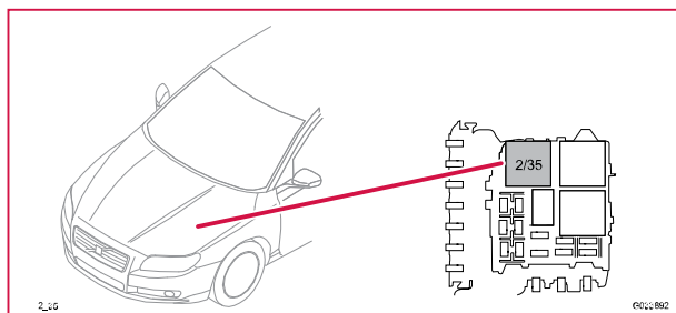
2/35 Relä startmotor
