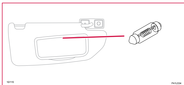
10/115 Lampa makeupspegel, höger solskydd
