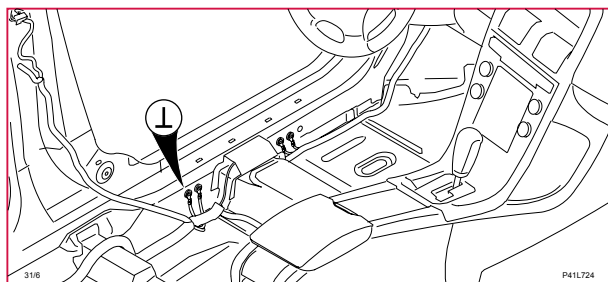
31/6 Stomanslutning, A-stolpe, förarsida
