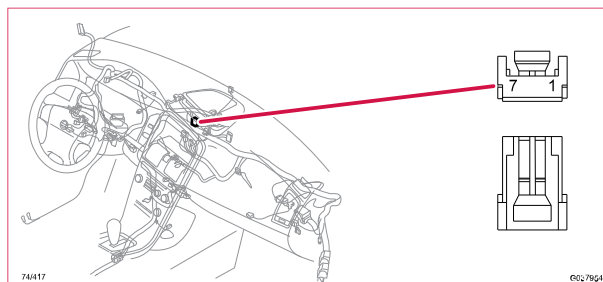
74/417 Kontaktstycke, GN
