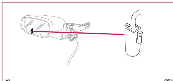
7/69 Givare, yttertemperatur
