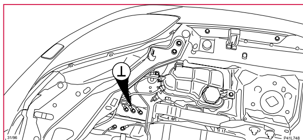
31/96 Stomanslutning, höger hjulhus 3
