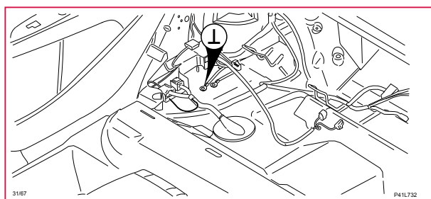
31/67 Stomanslutning, bakre sätesresare höger sida 1
