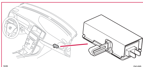
10/29 Handskfacksbelysning
