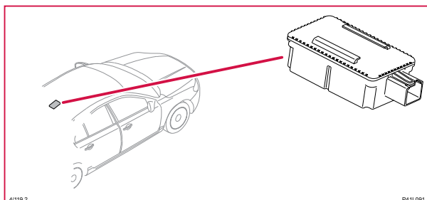
4/119.2 Fjärrmottagare (RRX)
