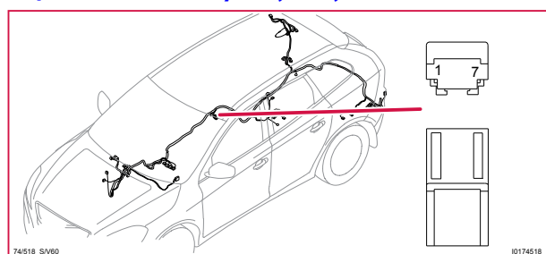
74/518 Kontaktstycke, GN, FOUR-C
