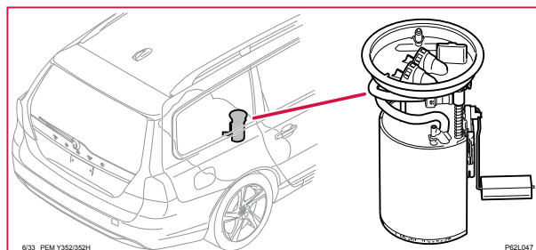
6/33 Bränslepump, V60H
