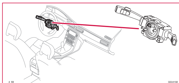
4/68 Styrenhet rattvinkelgivare (SAS)
