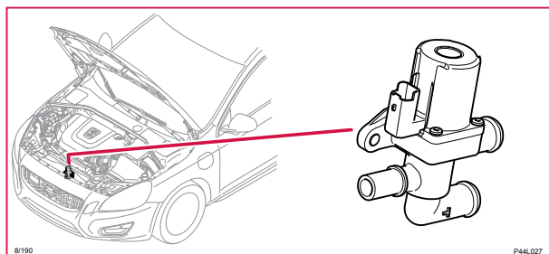
8/190 Ventil batterikylning 2
