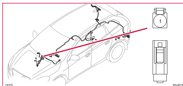
74/419 Kontaktstycke, BU
