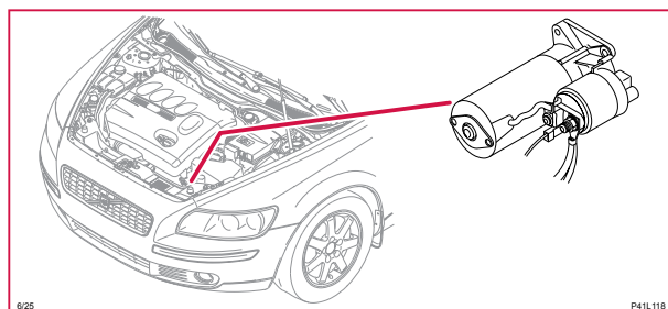
6/25 Startmotor
