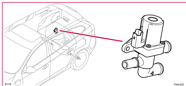
8/178 Avstängningsventil batterikylning
