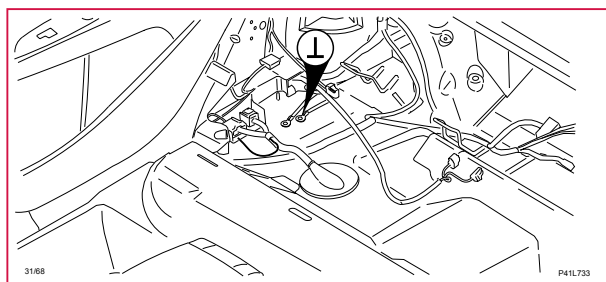
31/68 Stomanslutning, bakre sätesresare höger sida 2
