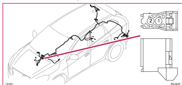
74/404 Kontaktstycke, BK
