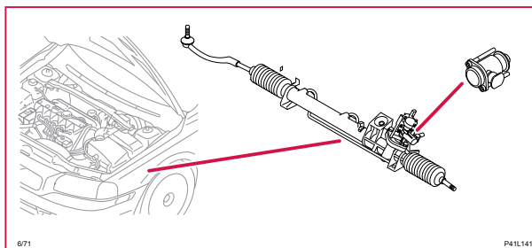
6/71 Ventil hastighetsberoende servostyrning
