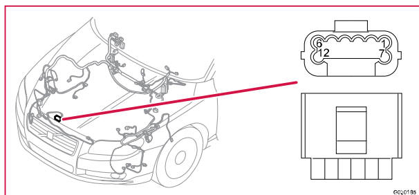
74/309 Kontaktstycke, GY
