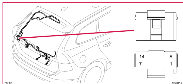
74/602 Kontaktstycke, GY, V60H
