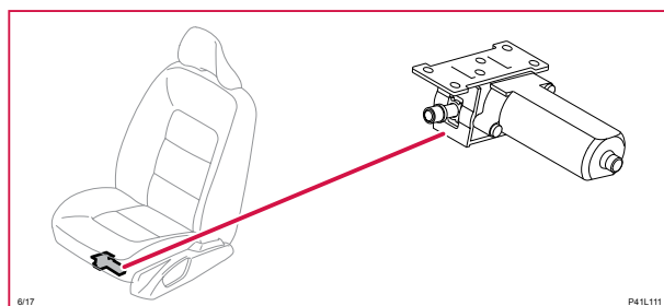
6/17 Säteslutningsmotor, förarsida
