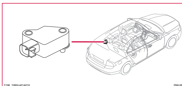
7/108 Sidokrockgivare bak vänster, S60LH
