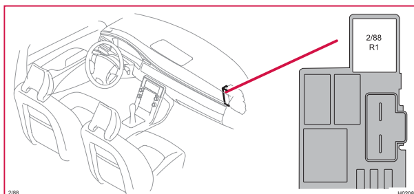
2/88 Relä 15-matning bak
