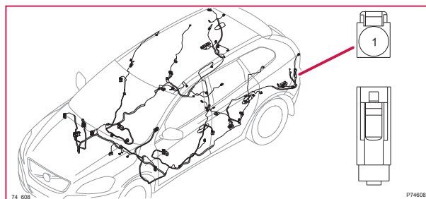
74/608 Kontaktstycke, WH, V60H
