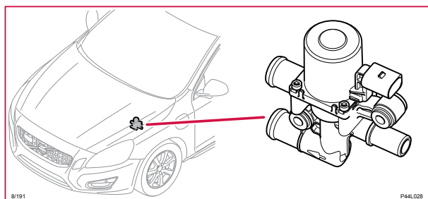
8/191 Parkeringsvärmarventil
