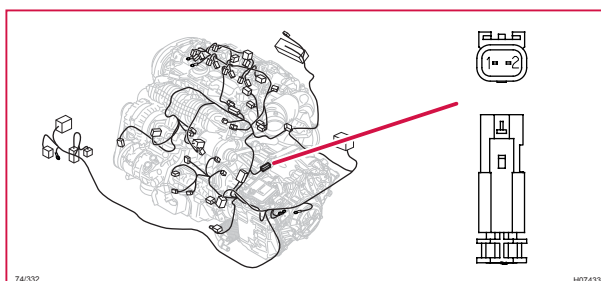
74/332 Kontaktstycke, BK, S60LH
