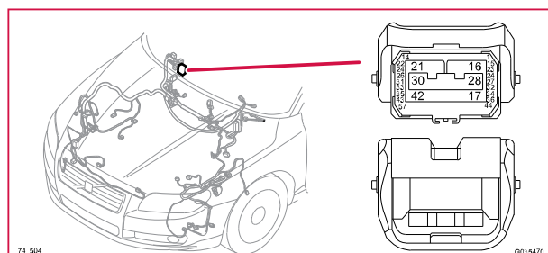
74/504 Kontaktstycke, WH
