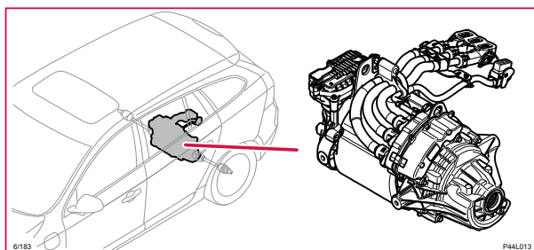
6/183 Elektrisk bakaxel ERAD
