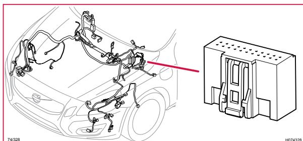
74/328 Kontaktstycke, GY, LHD
