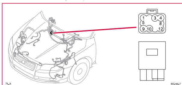
74/9 Kontaktstycke, BK
