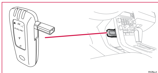
7/238 Givare alkoholås
