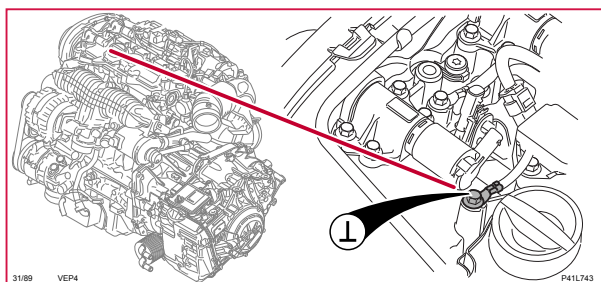
31/89 Stomanslutning, motor tändspolar
