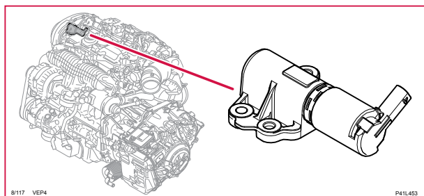
8/117 Solenoid variabel ventiltid, insugssida, S60LH
