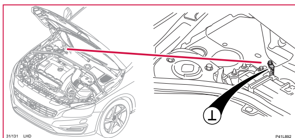
31/131 Stomanslutning, sekundärbatteri, LHD
