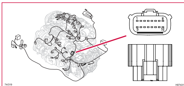
74/319 Kontaktstycke, BK, S60LH
