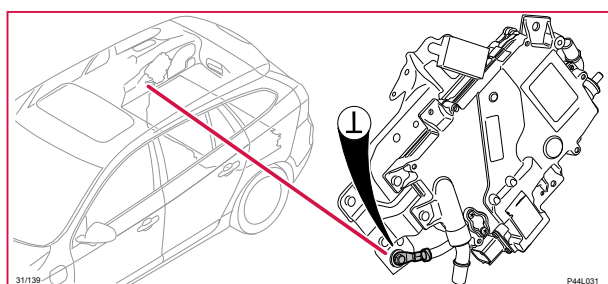
31/139 Stomanslutning, konsol DC/DC omvandlare
