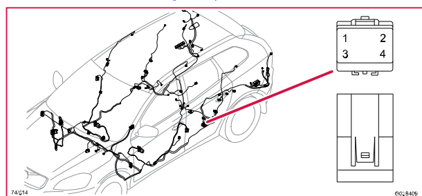
74/514 Kontaktstycke, GY
