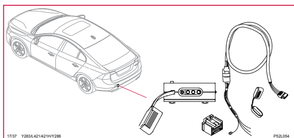
17/37 Uttag 4-poligt, ledningsmatta dragkrok, S60LH
