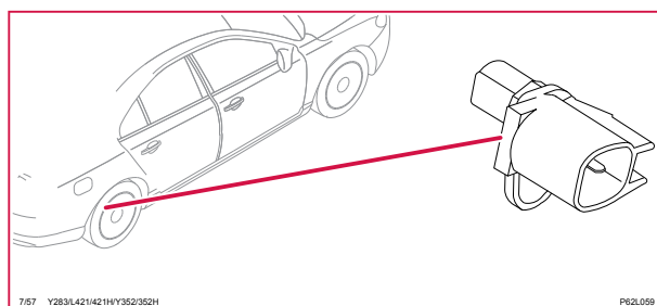
7/57 Givare, ABS, bakre höger
