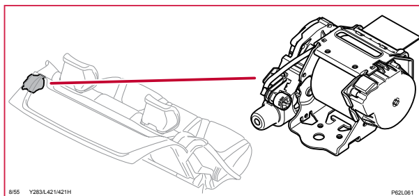
8/55 Tändare bältessträckare bak vänster, S60LH
