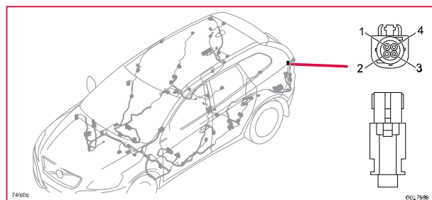
74/606 Kontaktstycke, BK, V60H & PAC
