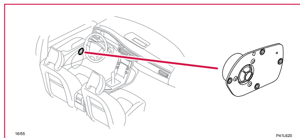
16/55 Högtalare, diskant, vänster framdörr
