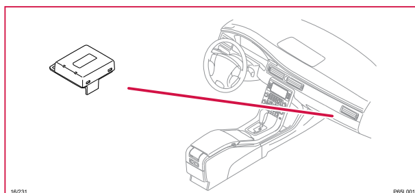
16/231 GNSS-antenn
