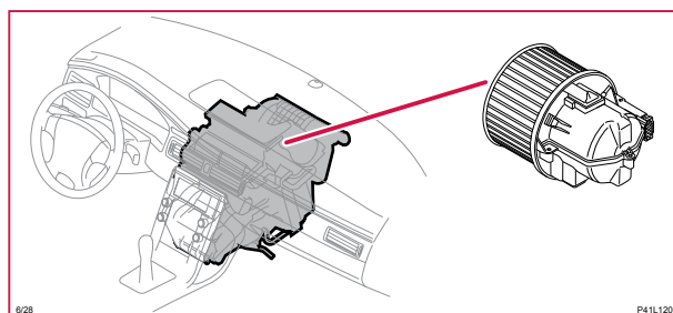
6/28 Motor kupéfläkt
