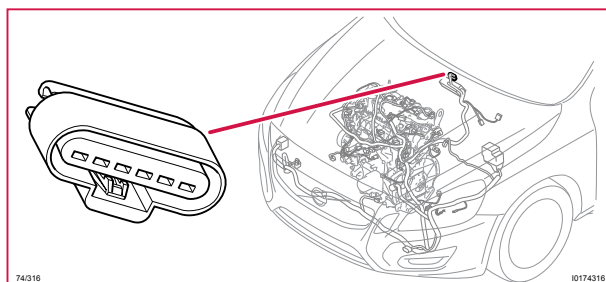
74/316 Kontaktstycke, BK
