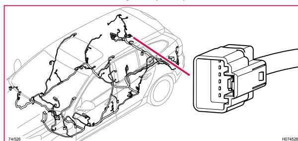
74/526 Kontaktstycke, GY, V60H
