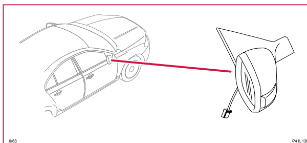
6/63 Motor, backspegel höger
