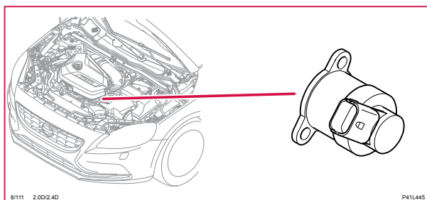
8/111 Reglerventil, bränsleflöde
