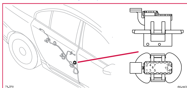
74/510 Kontaktstycke, BK
