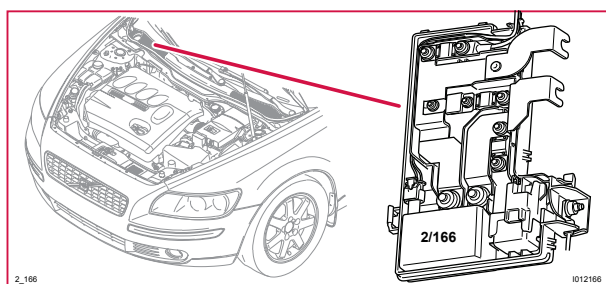
2/166 Batterirelä
