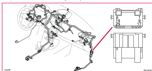
74/409 Kontaktstycke, GN
