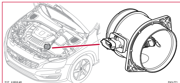
7/17 Luftmassmätare (MAF), V60H
