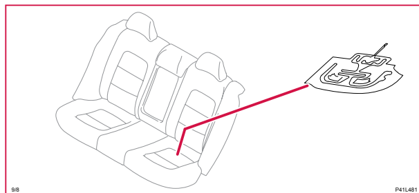
9/8 Värmeelement, vänster baksätesdyna
