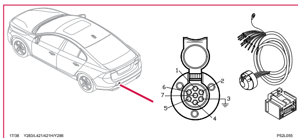
17/38 Uttag 7-poligt, ledningsmatta dragkrok, S60LH
