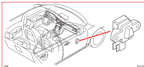
7/209 Sidokrockgivare, höger framdörr
