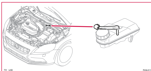
7/4 Givare bromsvätskenivå, LHD
