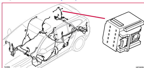
74/559 Kontaktstycke, GY
