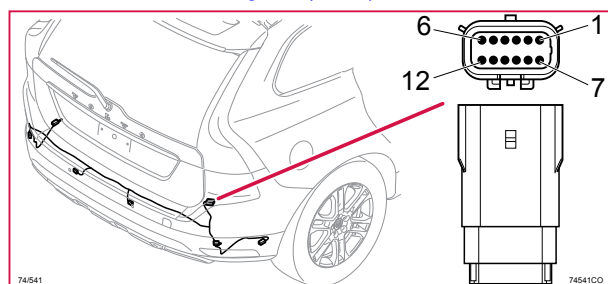
74/541 Kontaktstycke, BK, S60LH
