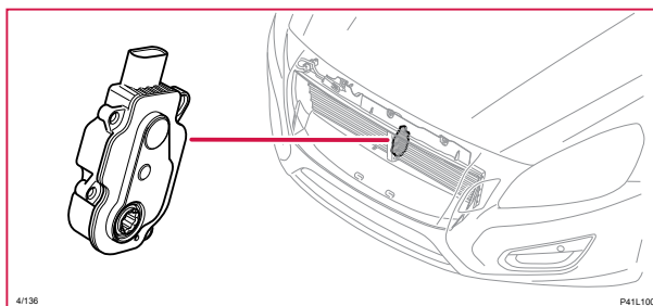
4/136 Styrenhet aktivt grillspjäll (AGM), V60H
