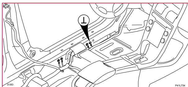
31/83 Stomanslutning, A-stolpe, förarsida
