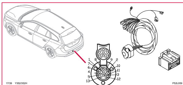
17/39 Uttag 13-poligt, ledningsmatta dragkrok, V60H
