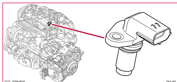
7/172 Lägesgivare kamaxel, insugssida, S60LH
