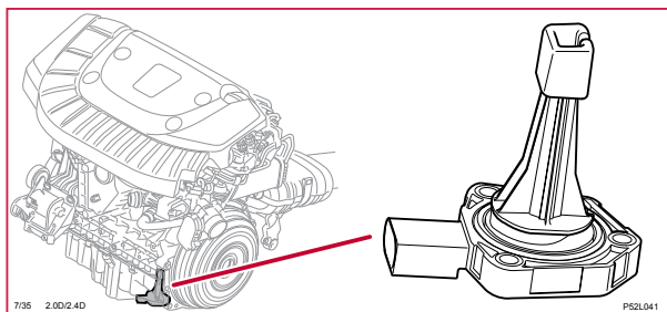
7/35 Givare oljenivå, V60H
