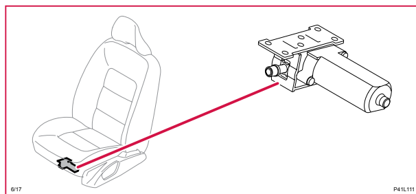
6/17 Säteslutningsmotor, förarsida
