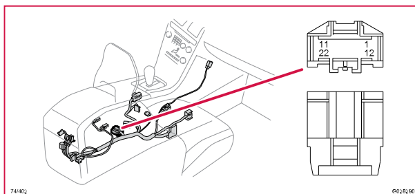
74/403 Kontaktstycke, GY
