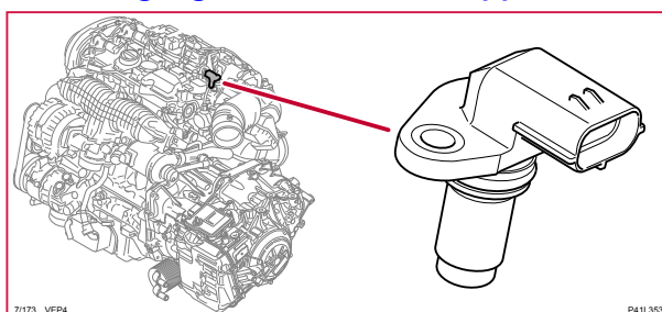
7/173 Lägesgivare kamaxel utloppssida
