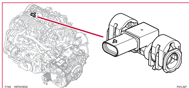
7/140 Bränsletryckgivare låg
