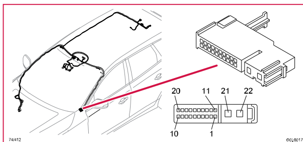
74/412 Kontaktstycke, GY
