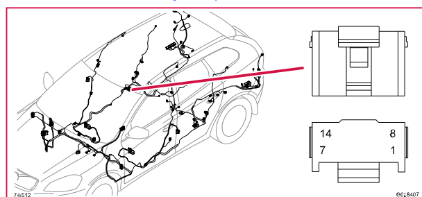
74/512 Kontaktstycke, GY
