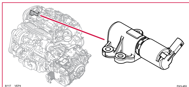
8/117 Solenoid variabel ventiltid, insugssida
