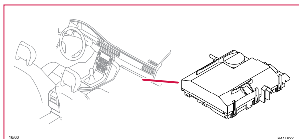
16/60 Telefonstyrenhet (PHM)
