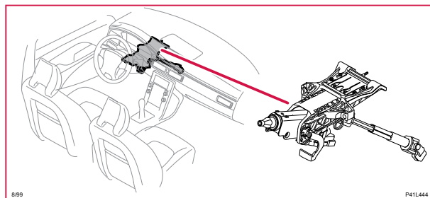
8/99 Tändare styrkolonn
