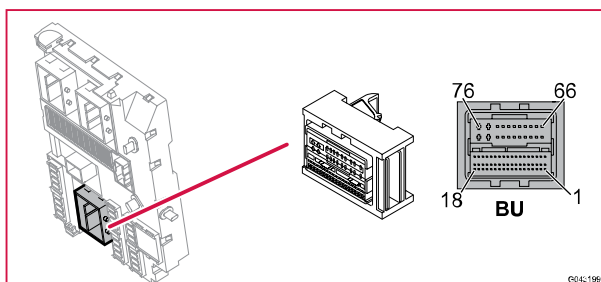
4/56:C3 Central elektronikstyrenhet (CEM)
