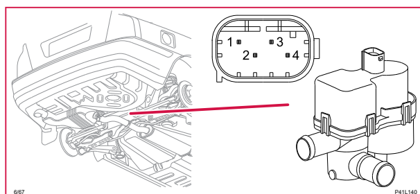
6/67 Pump bränsleläckagekontroll
