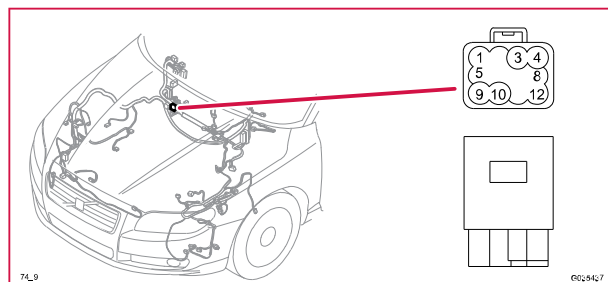
74/9 Kontaktstycke, BK, HEAT
