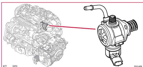
8/77 Reglerventil bränslevolym
