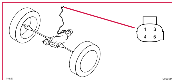
74/520 Kontaktstycke, GY, 4WD
