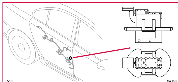
74/510 Kontaktstycke, BK
