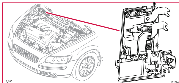
2/246 Relä, sekundärbatteri
