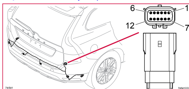
74/541 Kontaktstycke, GY
