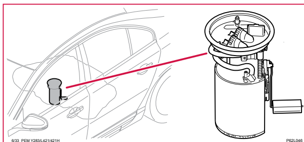
6/33 Bränslepump
