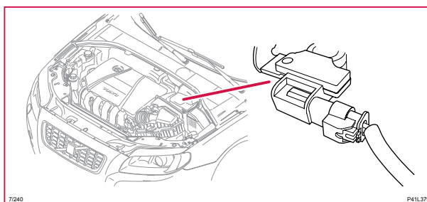
7/240 Batteriövervakningssensor (BMS)
