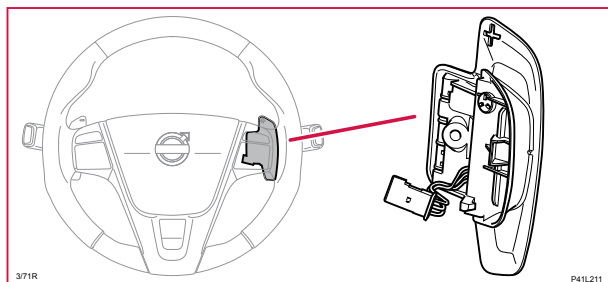
3/72 Växlingspaddel, höger
