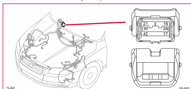
74/504 Kontaktstykke, WH
