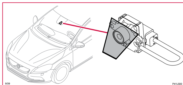
9/39 Värmeelement kamera
