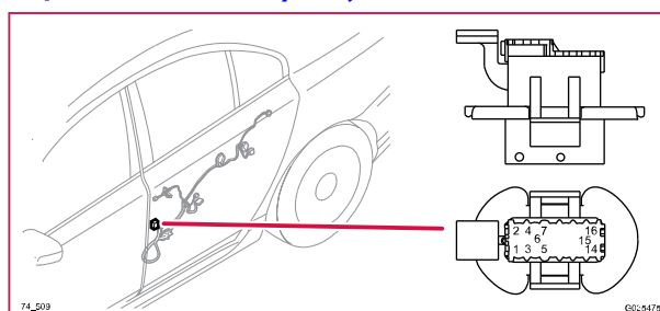
74/509 Kontaktstykke, BK
