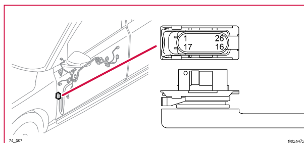
74/507 Kontaktstykke, BK
