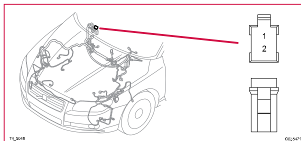
74/504B Kontaktstykke, BK
