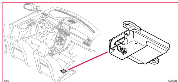
7/93 Passagerarviktsgivare (OWS)
