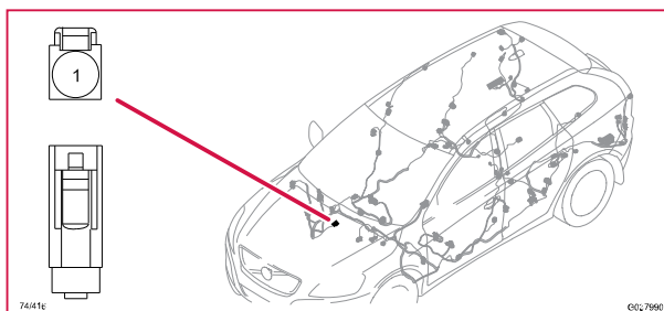
74/416 Kontaktstycke, VT
