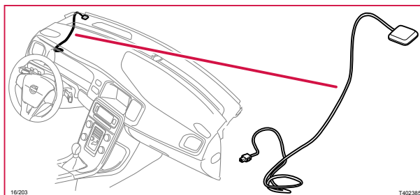
16/203 DSRC-antenn
