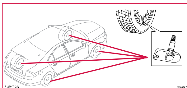
7/210-213 Däcktrycksgivare
