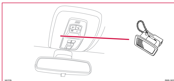
16/229 Reservmikrofon telematikmodul
