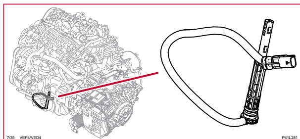
7/35 Givare oljenivå
