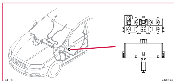
74/30 Kontaktstycke, BK
