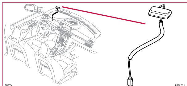
16/204 VICS-antenn
