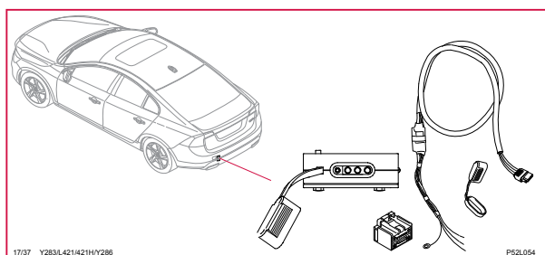
17/37 Uttag 4-poligt, ledningsmatta dragkrok
