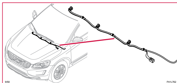
9/58 Uppvärmd vindruta spolarmunstycken
