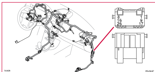
74/409 Kontaktstycke, GN
