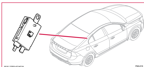
16/16 Förstärkare rutantenn
