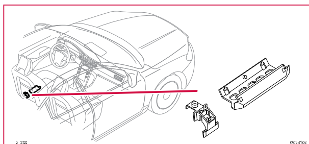
3/255 Lägesgivare förarsäte
