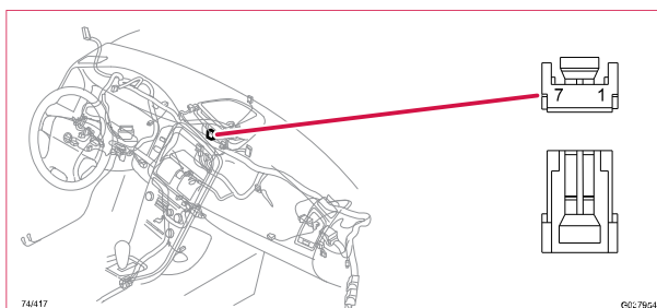
74/417 Kontaktstycke, GN
