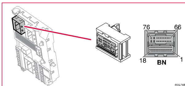
4/56:C2 Central elektronikstyrenhet (CEM)
