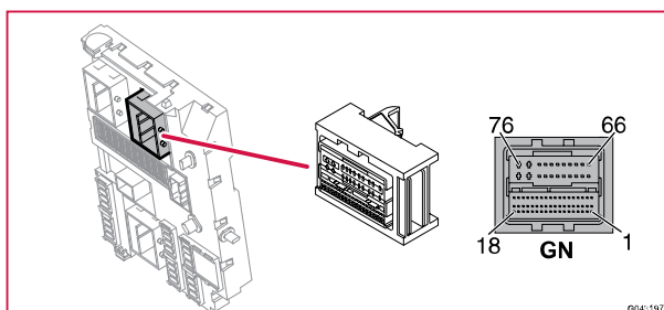
4/56:C1 Central elektronikstyrenhet (CEM)
