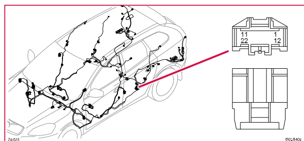
74/511 Kontaktstycke, GY
