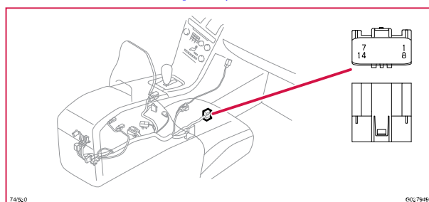
74/530 Kontaktstycke, GY
