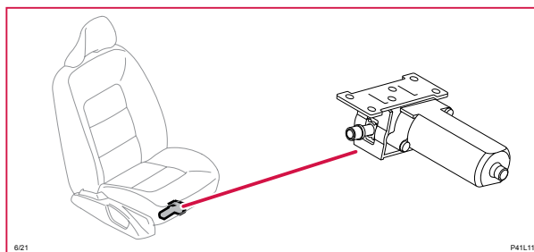
6/21 Säteslutningsmotor, passagerarsida
