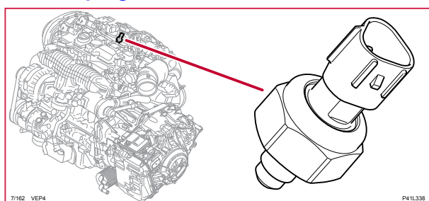
7/162 Tryckgivare bränslerör
