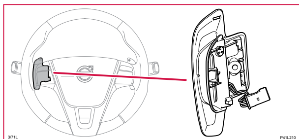
3/71 Växlingspaddel, vänster
