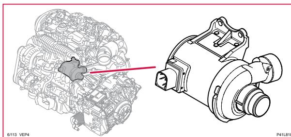
6/113 Kylvattenpump
