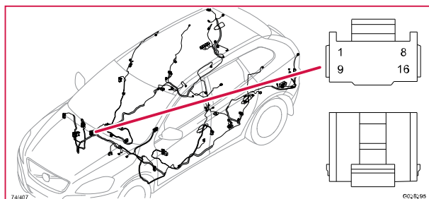
74/407 Kontaktstycke, GN
