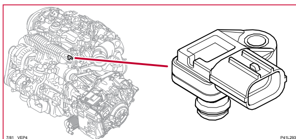
7/81 Tryckgivare inloppsrör
