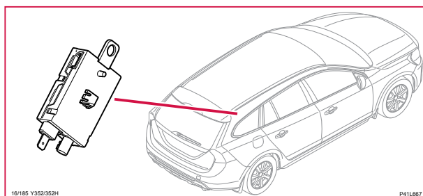
16/185 TV-Antenn, V60H
