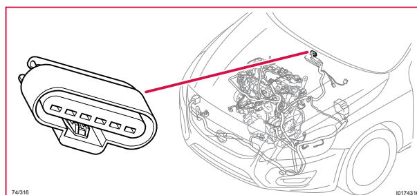
74/316 Kontaktstykke, BK
