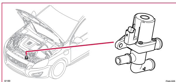
8/189 Ventil batterikylning 1
