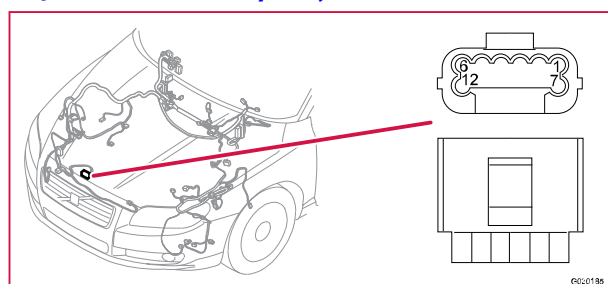
74/309 Kontaktstykke, GY
