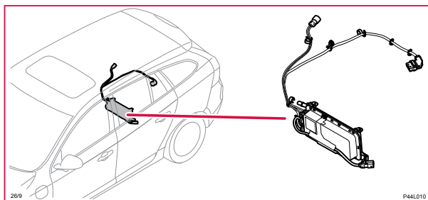
26/9 Batteriladdare (OBC)
