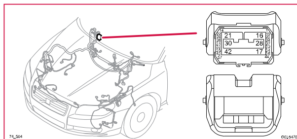
74/504 Kontaktstykke, WH
