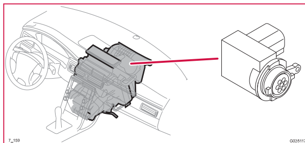
7/159 Luftkvalitetsgivare (AQS)
