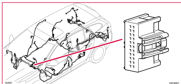
74/557 Kontaktstycke, GY
