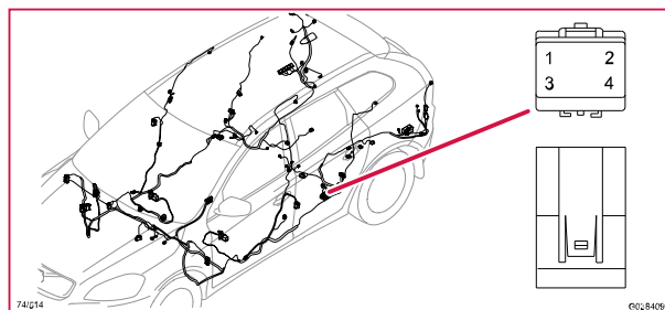
74/514 Kontaktstycke, GY
