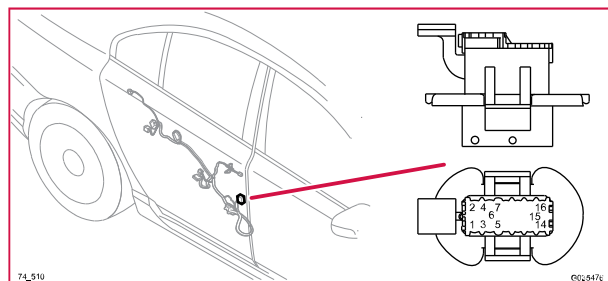
74/510 Kontaktstycke, BK
