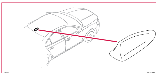
16/47 Antenn GSM/GPS/RDAR
