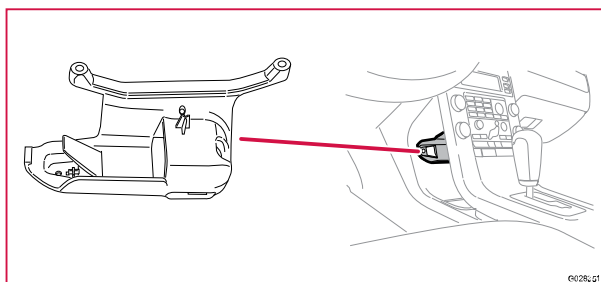
26/8 Laddningsvagg alkoholås
