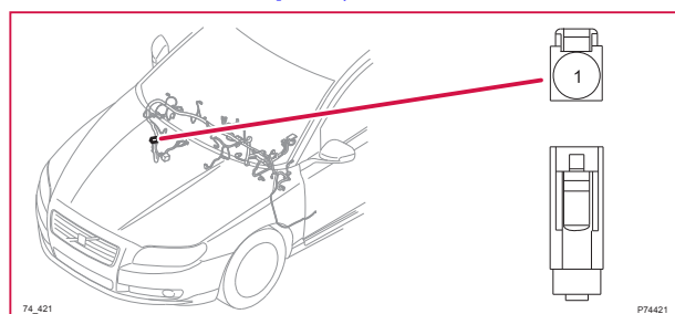
74/421 Kontaktstykke, GY
