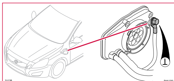
31/138 Skyddsjord laddanslutning
