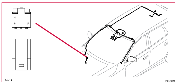
74/414 Kontaktstycke, BK
