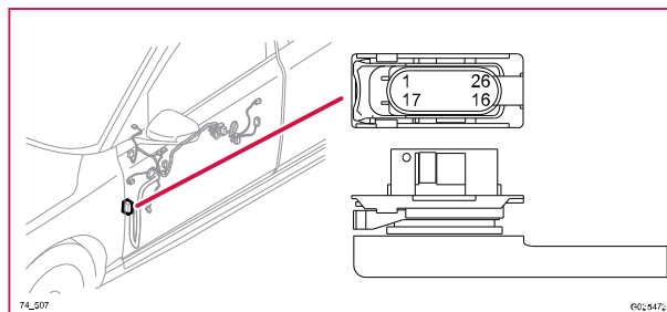
74/507 Kontaktstycke, BK
