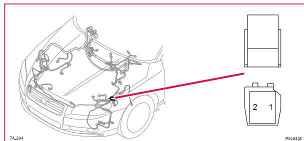
74/304 Kontaktstykke, BK, HEATNOZZ
