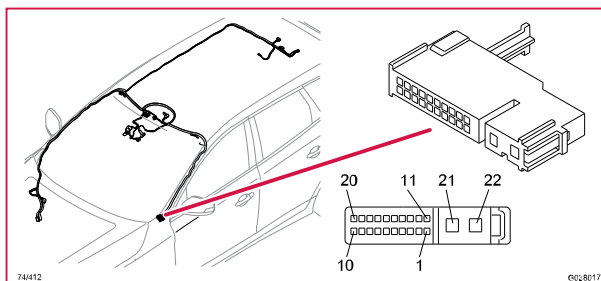
74/412 Kontaktstycke, GY
