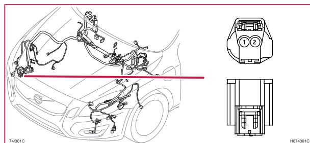
74/301C Kontaktstykke, GY, V60H
