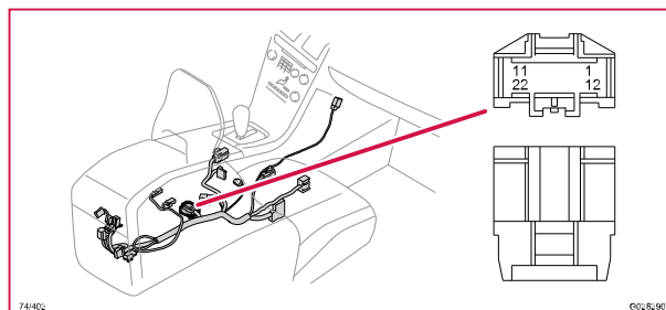
74/403 Kontaktstycke, GY
