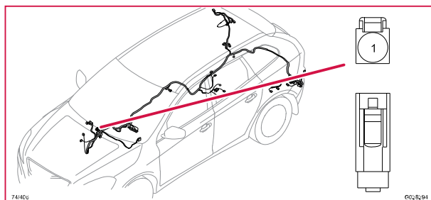
74/406 Kontaktstycke, VT
