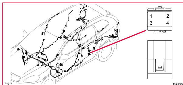
74/514 Kontaktstycke, GY
