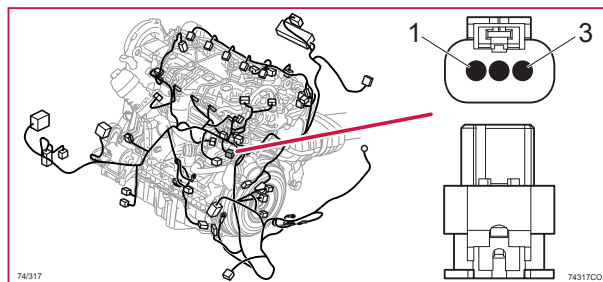
74/317 Kontaktstykke, BK
