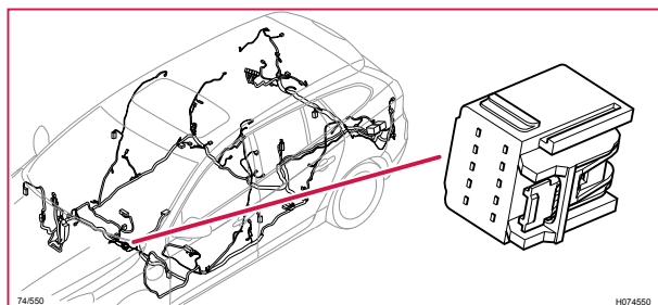
74/550 Kontaktstycke, GY
