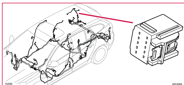
74/559 Kontaktstycke, GY
