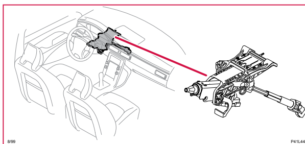
8/99 Tändare styrkolonn
