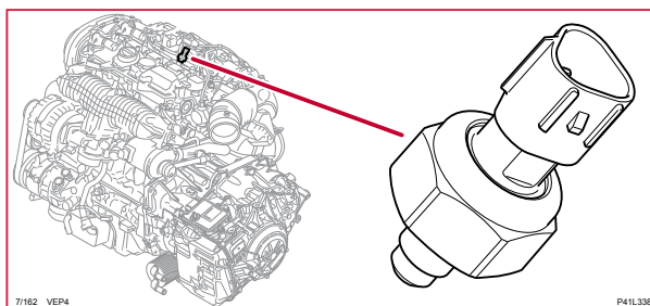
7/162 Tryckgivare bränslerör, S60LH
