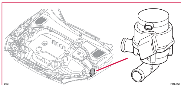
6/73 Kylvätskepump
