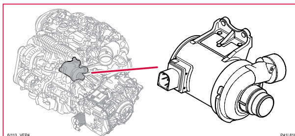
6/113 Kylvattenpump, S60LH
