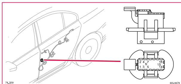
74/509 Kontaktstycke, BK
