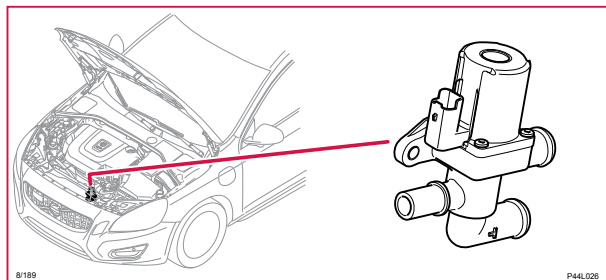
8/189 Ventil batterikylning 1
