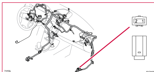
74/405 Kontaktstycke, WH
