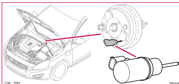
7/160 Bromsvakuumbgivare
