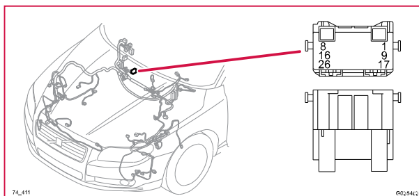
74/411 Kontaktstycke, GY
