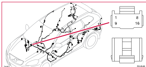
74/407 Kontaktstycke, GN
