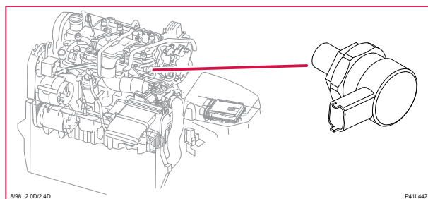
8/98 Reglerventil bränsletryck
