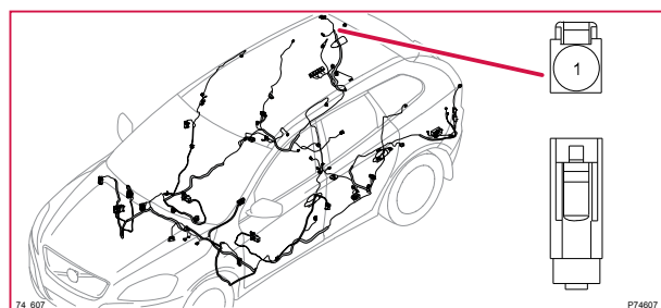
74/607 Kontaktstycke, BK, V60
