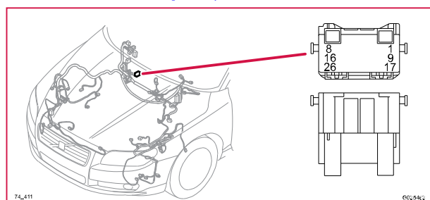
74/411 Kontaktstycke, GY
