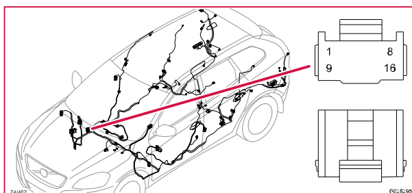
74/407 Kontaktstycke, GN
