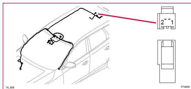
74/609 Kontaktstycke, GY, V60
