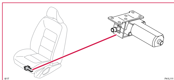
6/17 Sätesslutningsmotor, förarsida
