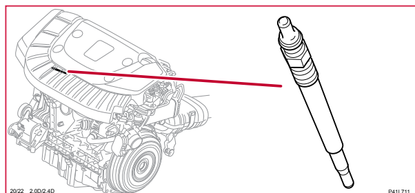
20/22-26 Glödstift, D
