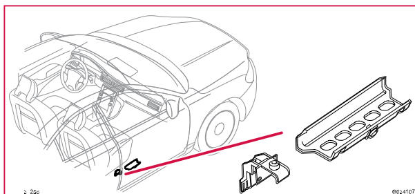
3/256 Lägesgivare passagerarstol
