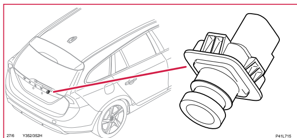
27/6 Kamera, V60
