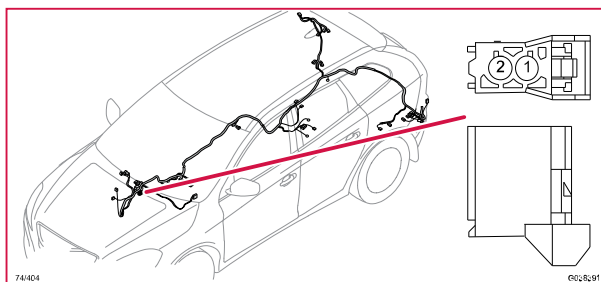
74/404 Kontaktstycke, BK
