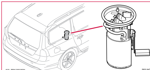
6/33 Bränslepump, V60
