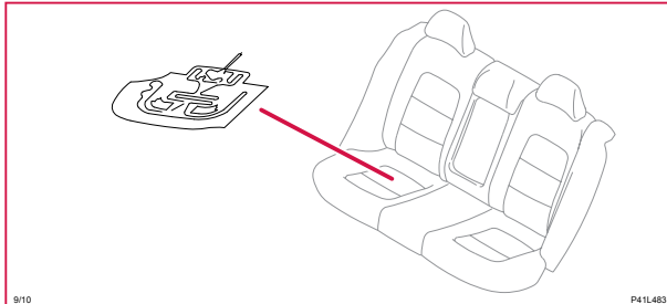
9/10 Värmeelement, höger baksätessdyna
