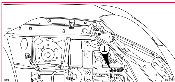
31/4 Stomanslutning, Motor
