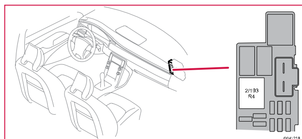
2/193 Relä komfortfunktioner
