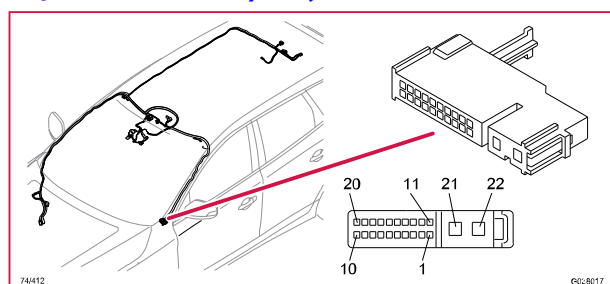
74/412 Kontaktstycke, GY
