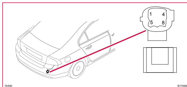
74/540 Kontaktstycke, GY
