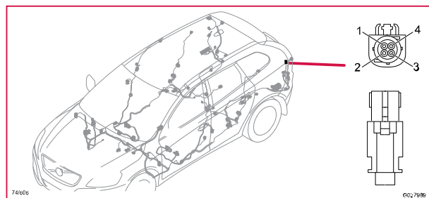
74/606 Kontaktstycke, BK
