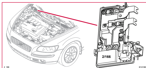
2/166 Batterirelä
