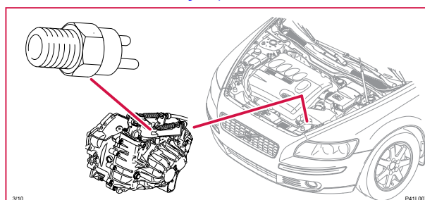
3/10 Kontakt backljus, MAN
