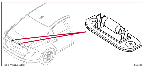
10/3 Skyltbelysning, S60
