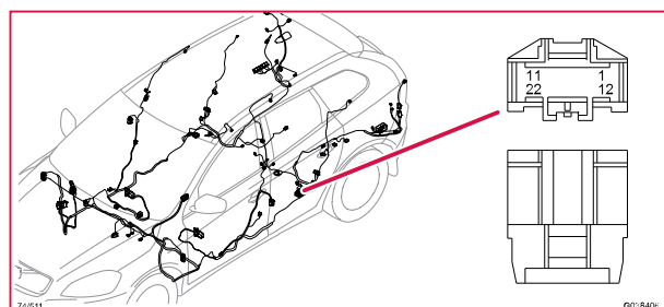
74/511 Kontaktstycke, GY
