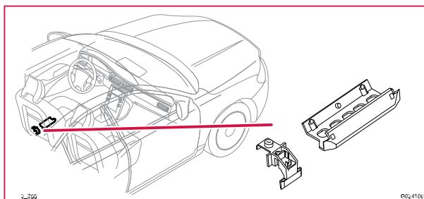
3/255 Lägesgivare förarsäte
