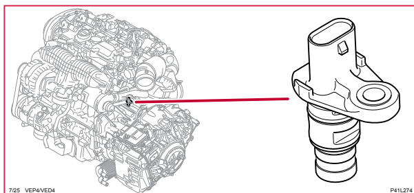
7/25 Impulsgivare, 4-CYL
