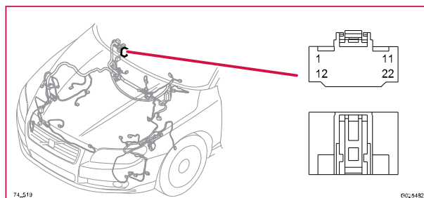
74/519 Kontaktstycke, GY
