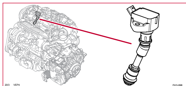
20/3-8 Tändstift med tändspolar, P
