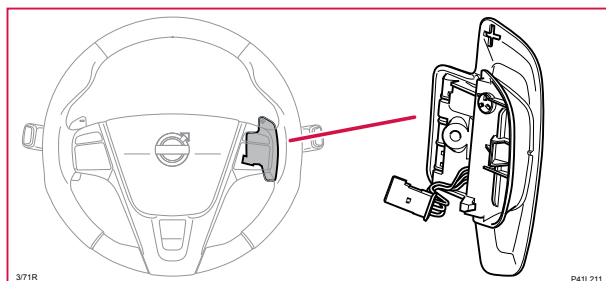
3/72 Växlingspaddel, höger
