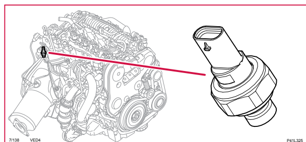
7/138 Avgasttryckgivare, 4-CYL D
