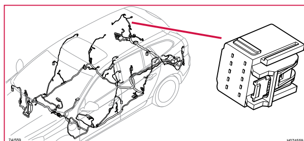
74/559 Kontaktstycke, GY
