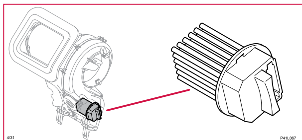
4/31 Fläktstyrenhet, kupé
