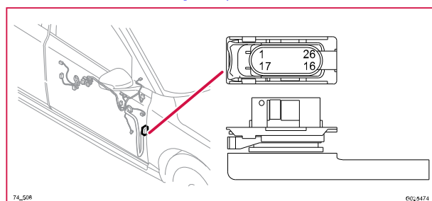
74/508 Kontaktstycke, BK
