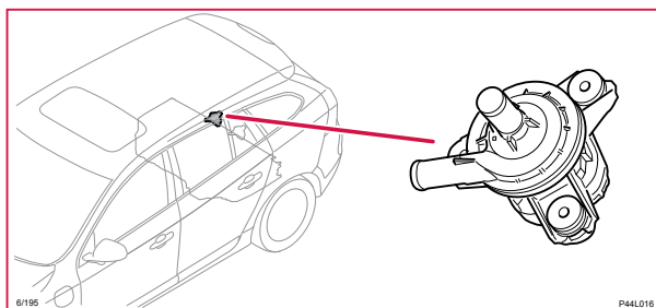
6/195 Batterikylvattenpump 1
