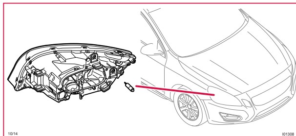
10/14 Körriktningsvisare fram höger
