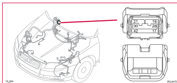
74/504 Kontaktstycke, WH
