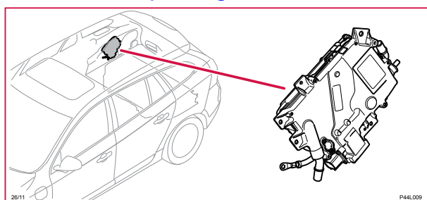
26/11 DC/DC spänningsomvandlare
