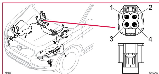
74/330 Kontaktstycke, GY
