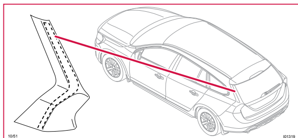
10/51 Bakljuslampa 1, vänster
