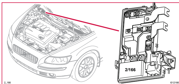
2/166 Batterirelä
