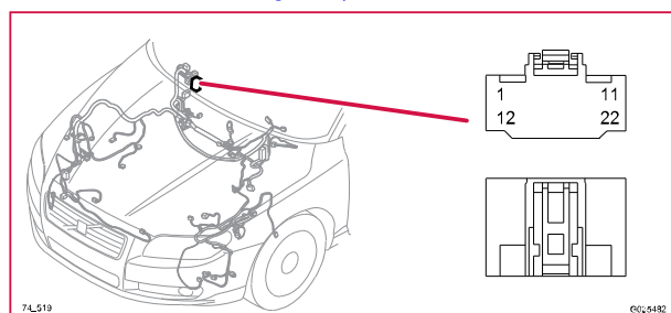
74/519 Kontaktstycke, GY
