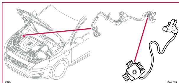
8/185 Klimatavstängningsventil
