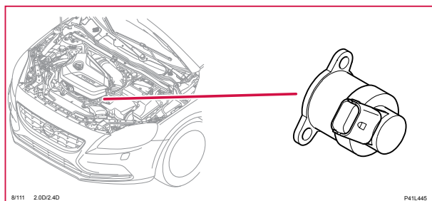
8/111 Reglerventil, bränsleflöde
