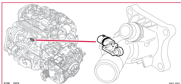
8/166 Elektrisk termostat, motorkylsystem, S60LH
