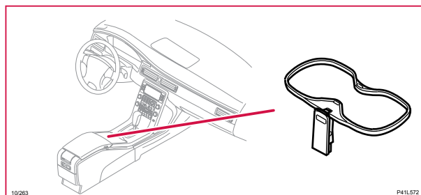
10/263 Tunnelkonsolsbelysning, mugghållare
