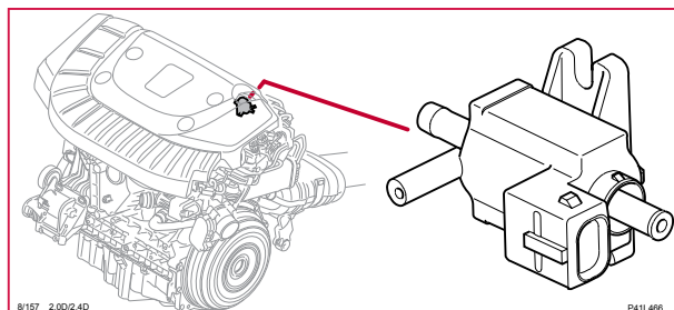
8/157 Turboreglerventil, V60H
