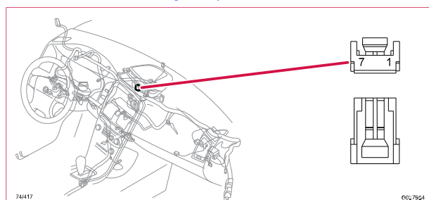
74/417 Kontaktstycke, GN
