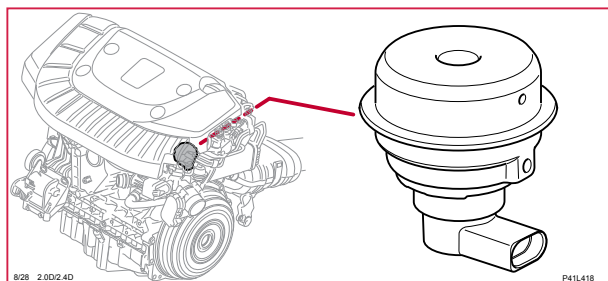
8/28 Turboreglerventil, V60H
