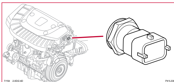
7/154 Givare bränsletemperatur, V60H
