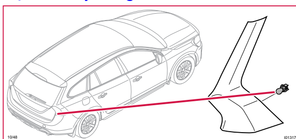
10/48 Backljus höger
