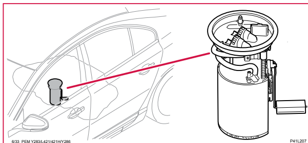
6/33 Bränslepump, S60LH
