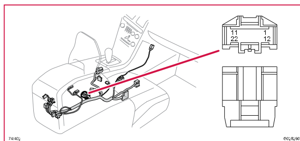
74/403 Kontaktstycke, GY
