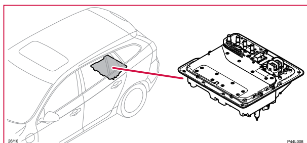
26/10 Spänningsomvandlingsenhet (ISC)
