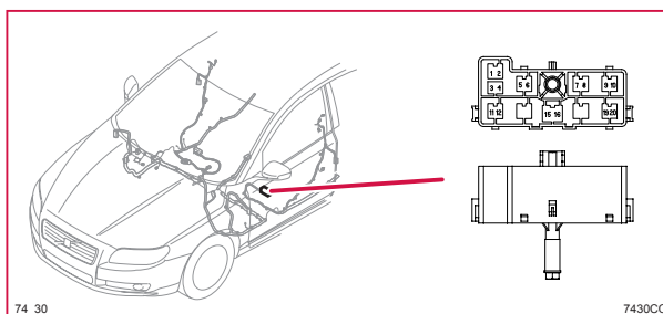
74/30 Kontaktstycke, BK
