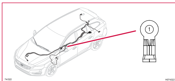
74/322 Kontaktstycke, V60H
