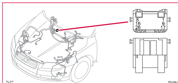
74/411 Kontaktstycke, GY
