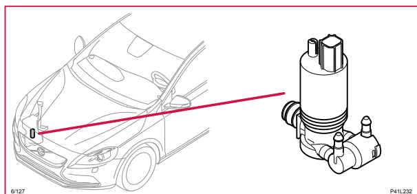
6/127 Spolarmotor
