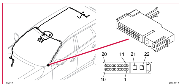
74/412 Kontaktstycke, GY
