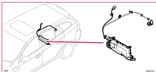
26/9 Batteriladdare (OBC)
