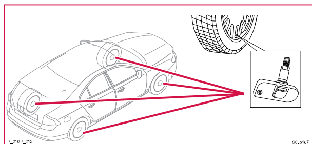
7/210-213 Däcktrycksgivare
