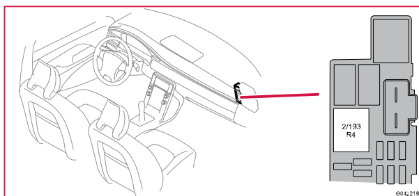
2/193 Relä komfortfunktioner
