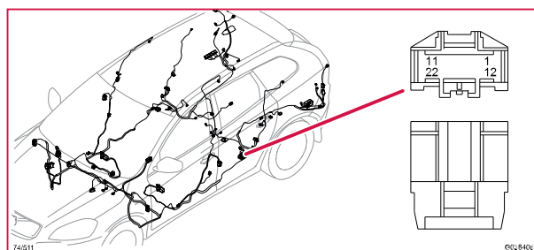
74/511 Kontaktstycke, GY
