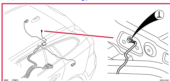
30/2 Stomanslutning, skena bakre
