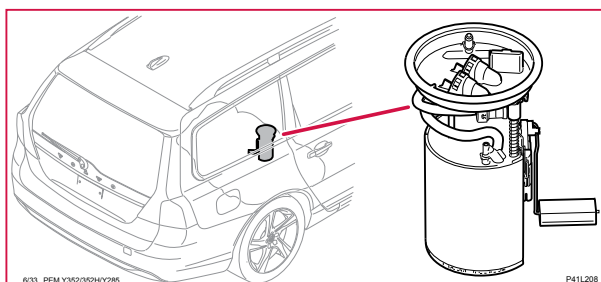
6/33 Bränslepump, V60H
