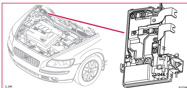
2/246 Relä, sekundärbatteri
