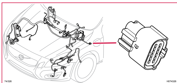
74/326 Kontaktstycke, BK
