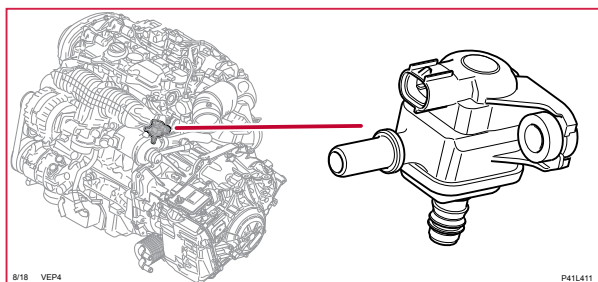
8/18 EVAP-ventil, S60LH
