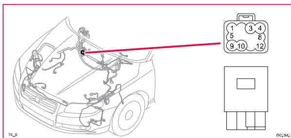
74/9 Kontaktstycke, BK
