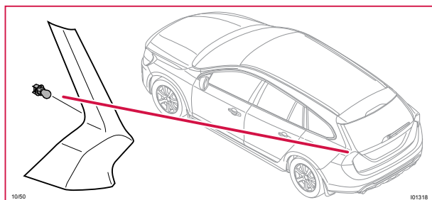
10/50 Bromsljus vänster
