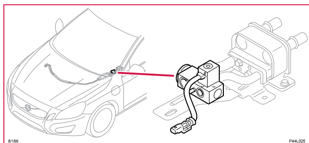
8/186 Avstängningsventil kylmedium
