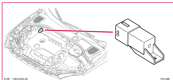
4/109 Styrenhet glödstift, V60H
