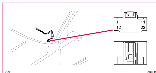
74/401 Kontaktstycke, GY
