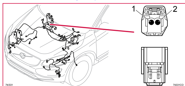
74/331 Kontaktstycke, BK
