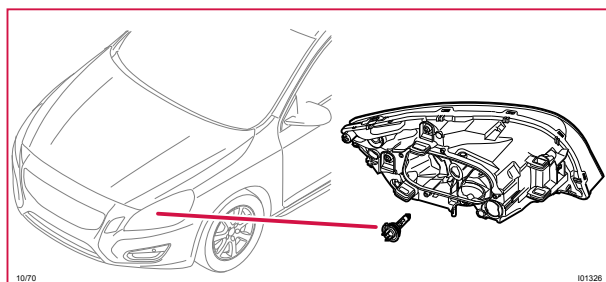
10/70 Halvljus vänster
