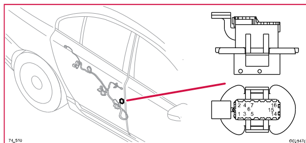
74/510 Kontaktstycke, BK
