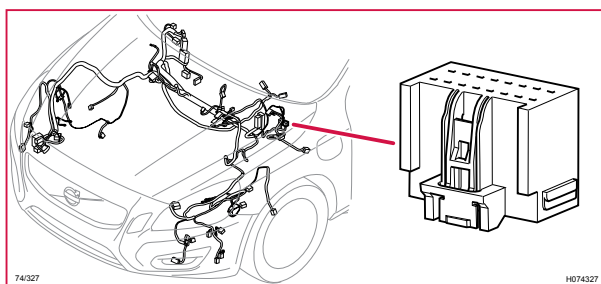
74/327 Kontaktstycke, GN
