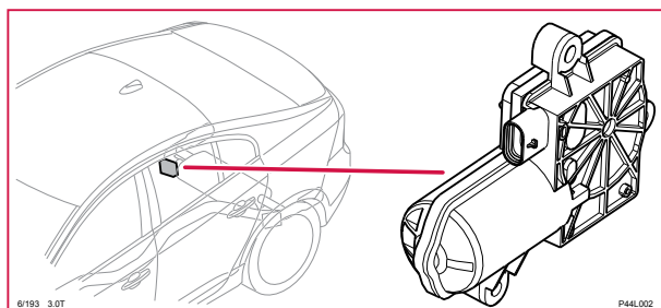
6/193 Avgasljud och effektregermotor, höger, S60LH
