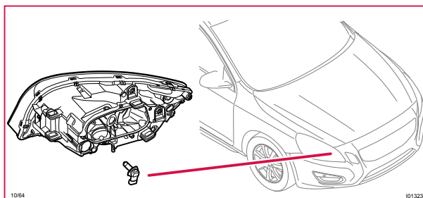
10/64 Helljus höger
