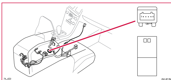
74/420 Kontaktstycke, GY
