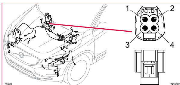
74/330 Kontaktstycke, GY
