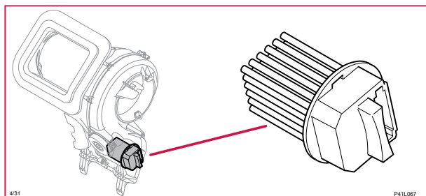
4/31 Fläktstyrenhet, kupé
