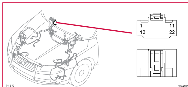
74/519 Kontaktstycke, GY
