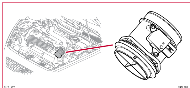
7/17 Luftmassmätare (MAF), 5-CYL P
