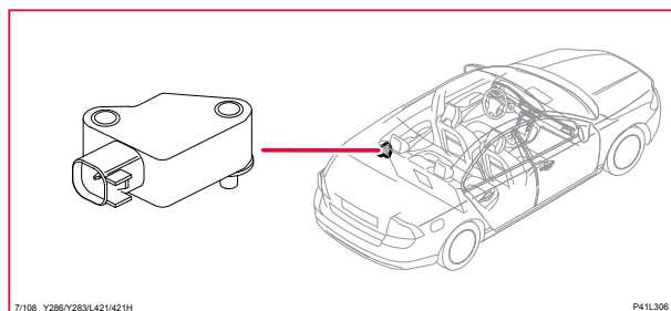
7/108 Sidokrockgivare bak vänster, S60
