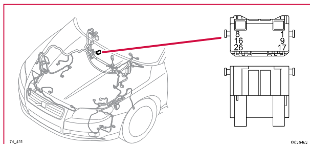
74/411 Kontaktstycke, GY
