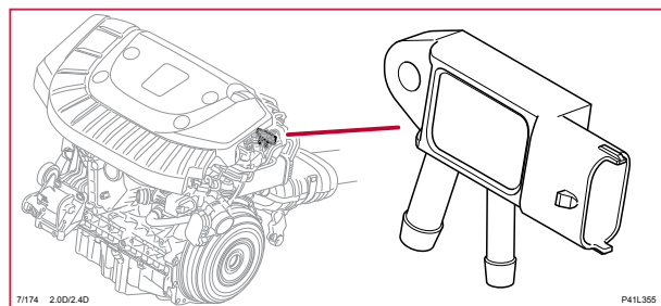
7/174 Tryckgivare, partikelfilter, 5-CYL D
