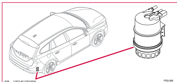
9/38 Eluppvärmt bränslefilter, V60 & 5-CYL D
