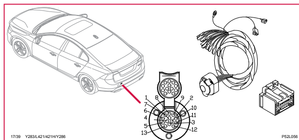
17/39 Uttag 13-poligt, ledningsmatta dragkrok, S60
