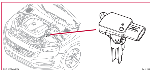
7/17 Luftmassmätare (MAF), 4-CYL
