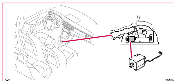
8/36 Solenoid, växlingsspärr
