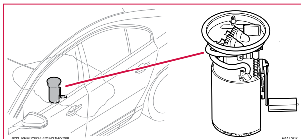
6/33 Bränslepump, S60
