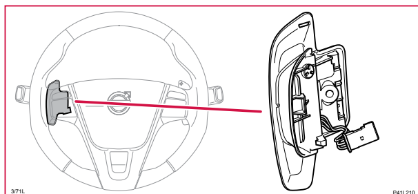
3/71 Växlingspaddel, vänster
