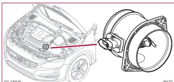
7/17 Luftmassmätare (MAF), 5-CYL D
