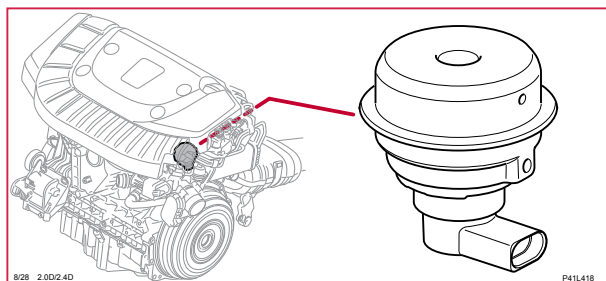
8/28 Turboreglerventil, 5-CYL D
