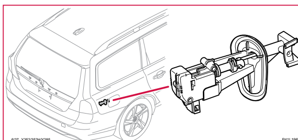
6/37 Låsmotor tanklucka, V60
