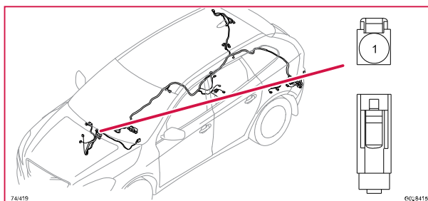
74/419 Kontaktstycke, BU
