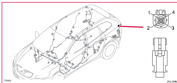
74/606 Kontaktstycke, BK
