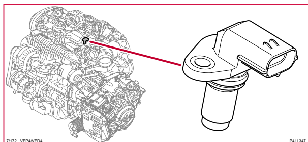
7/172 Lägesgivare kamaxel, insugssida, 4-CYL
