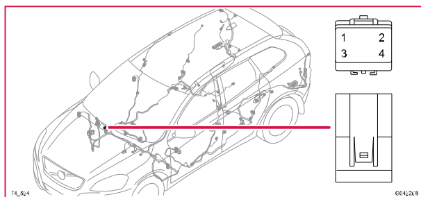
74/534 Kontaktstycke, GY
