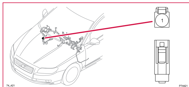
74/421 Kontaktstycke, GY
