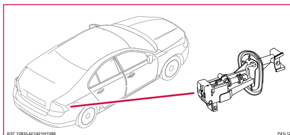
6/37 Låsmotor tanklucka, S60
