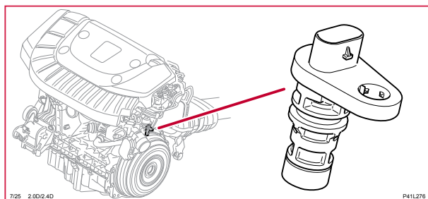
7/25 Impulsgivare, 5-CYL D
