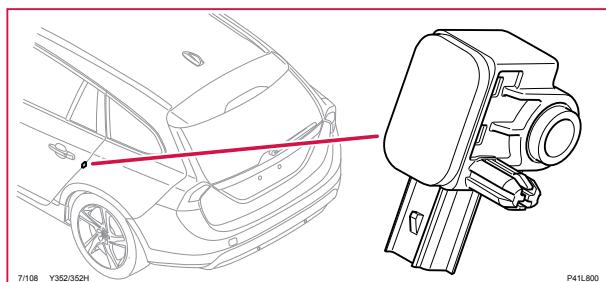
7/108 Sidokrockgivare bak vänster, V60
