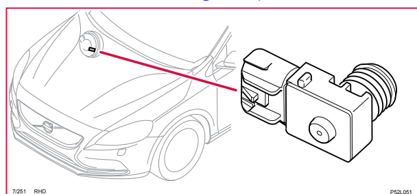
7/251 Bromsvakuumgivare, RHD
