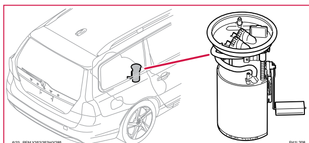
6/33 Bränslepump, V60
