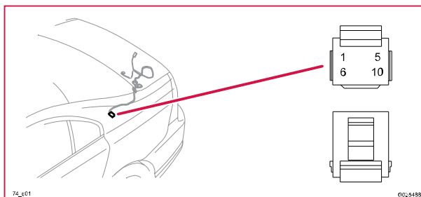
74/601 Kontaktstycke, GY, S60
