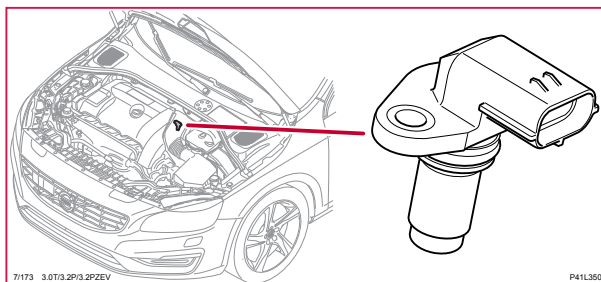
7/173 Lägesgivare kamaxel utloppssida, 6-CYL
