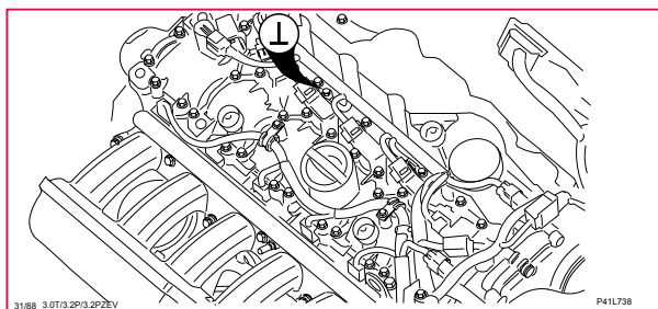
31/88 Stomanslutning, motor tändspolar, 6-CYL
