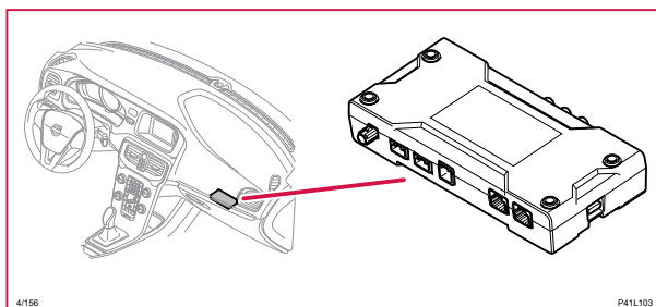
4/156 Uppkopplingsenhet tillbehör
