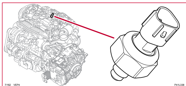
7/162 Tryckgivare bränslerör, 4-CYL P
