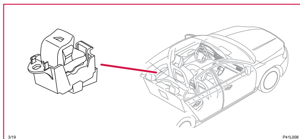
3/19 Omkopplare, elektriska fönsterhissar, vänster baddörr
