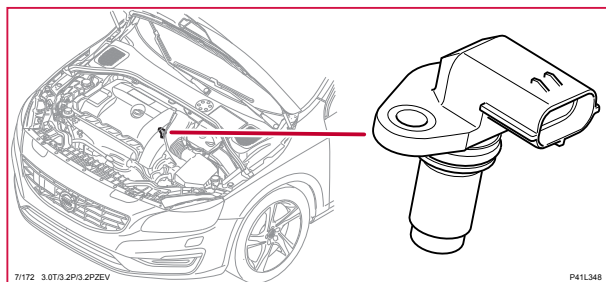
7/172 Lägesgivare kamaxel, insugssida, 6-CYL
