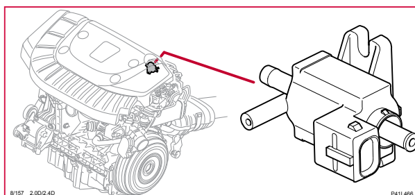
8/157 Turboreglerventil, 5-CYL D
