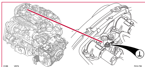
31/88 Stomanslutning, motor tändspolar, 4-CYL P
