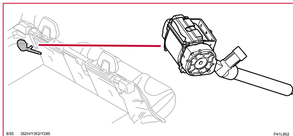
8/55 Tändare bältessträckare bak vänster, V60
