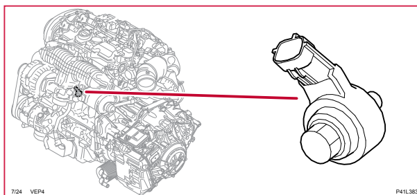
7/24 Knackgivare främre, 4-CYL P
