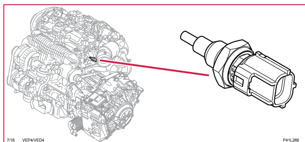
7/16 Givare kylvätsketemperatur, 4-CYL
