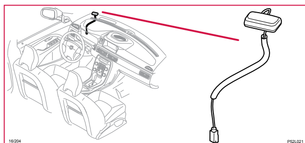
16/204 VICS-antenn
