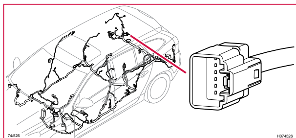
74/526 Kontaktstycke, GY
