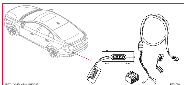
17/37 Uttag 4-poligt, ledningsmatta dragkrok, S60
