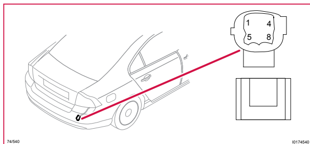
74/540 Kontaktstycke, GY
