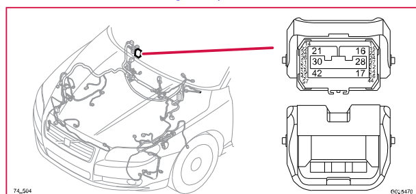
74/504 Kontaktstycke, WH
