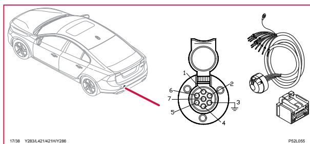
17/38 Uttag 7-poligt, ledningsmatta dragkrok, S60
