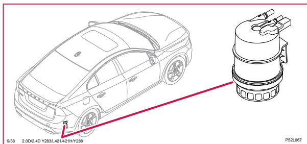
9/38 Eluppvärmt bränslefilter, S60 & 5-CYL D
