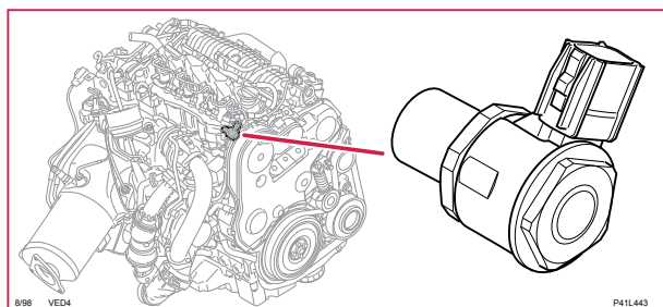
8/98 Reglerventil bränsletryck, 4-CYL D
