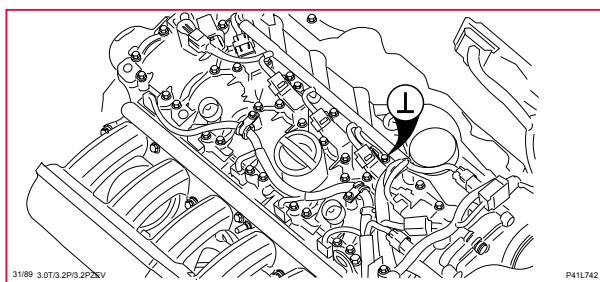
31/89 Stomanslutning, motor tändspolar, 6-CYL
