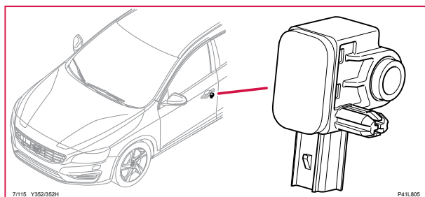
7/115 Sidokrockgivare vänster B-stolpe, V60
