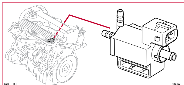
8/28 Turboreglerventil, 5-CYL P
