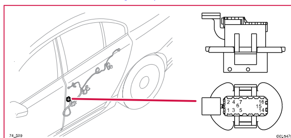
74/509 Kontaktstycke, BK
