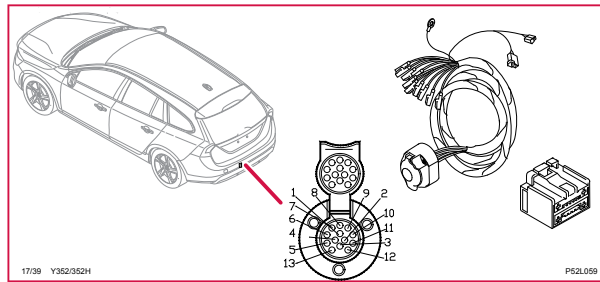
17/39 Uttag 13-poligt, ledningsmatta dragkrok, V60
