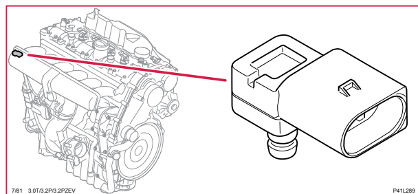
7/81 Tryckgivare inloppsrör, 6-CYL
