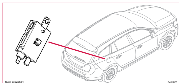
16/73 Förstärkare rutantenn 2 (TV/DAB), V60
