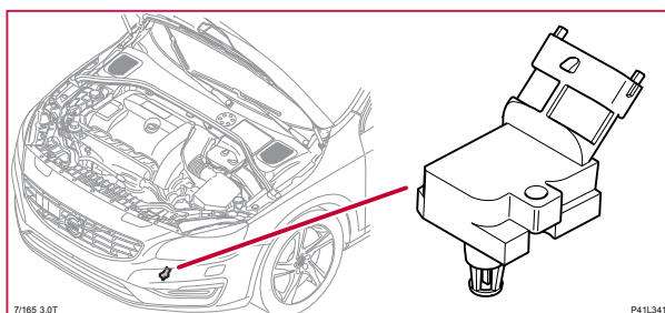
7/165 Tryck- och temperaturgivare inloppsrör, 6-CYL
