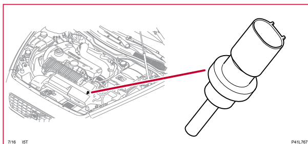
7/16 Givare kylvätsketemperatur, 5-CYL P
