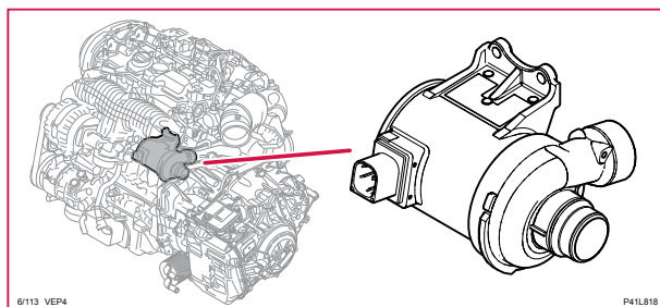
6/113 Kylvattenpump, 4-CYL P
