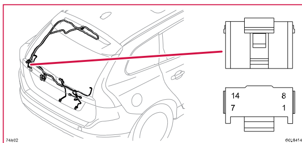
74/602 Kontaktstycke, GY, V60
