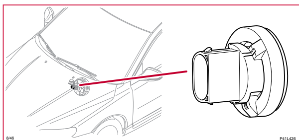
8/46 Aktiveringsenhet DSTC
