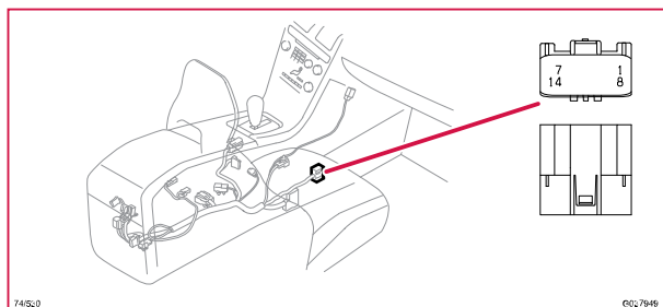
74/530 Kontaktstycke, GY
