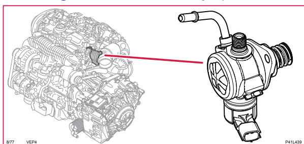
8/77 Reglerventil bränslevolym, 4-CYL P
