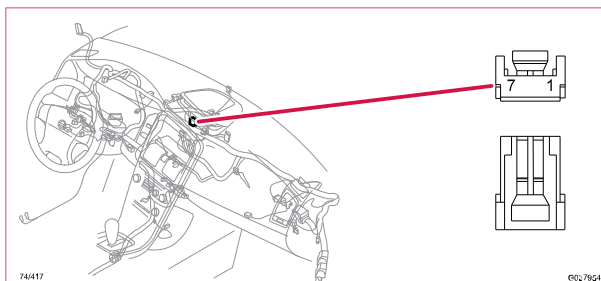
74/417 Kontaktstycke, GN
