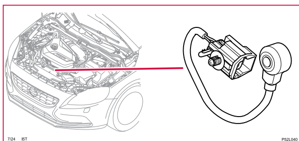
7/24 Knackgivare främre, 5-CYL P
