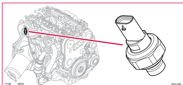
7/138 Avgastryckgivare, 4-CYL D
