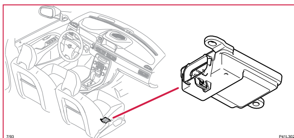
7/93 Passagerarviktsgivare (OWS)
