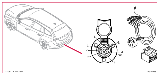
17/38 Uttag 7-poligt, ledningsmatta dragkrok, V60
