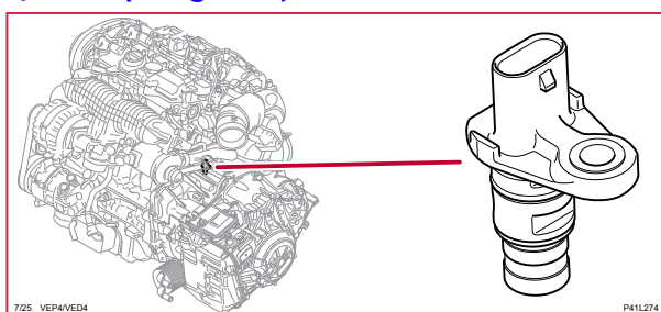
7/25 Impulsgivare, 4-CYL
