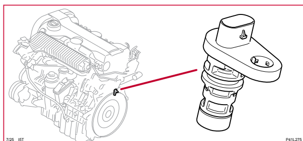
7/25 Impulsgivare, 5-CYL P
