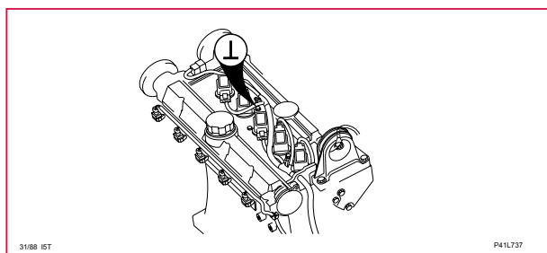
31/88 Stomanslutning, motor tändspolar, 5-CYL P
