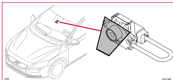
9/39 Värmeelement kamera
