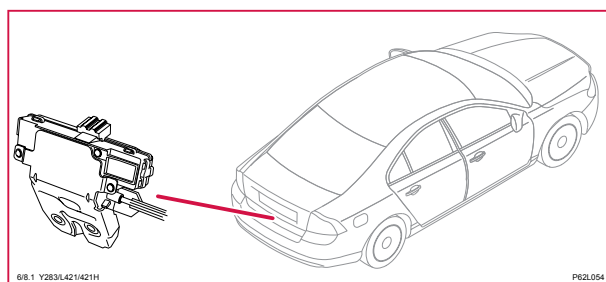
6/8 Centrallåsmotor, bagageutrymme, V60
