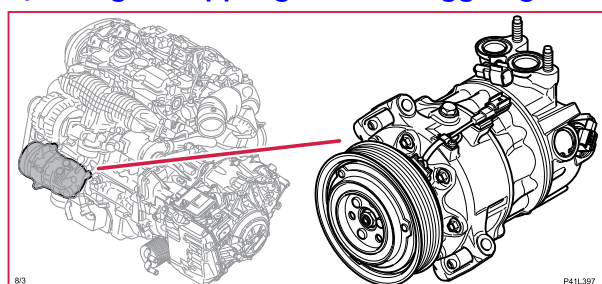
8/3 Magnetkoppling klimatanläggning
