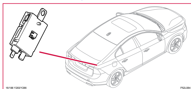
16/188 TV-Antenn, S60
