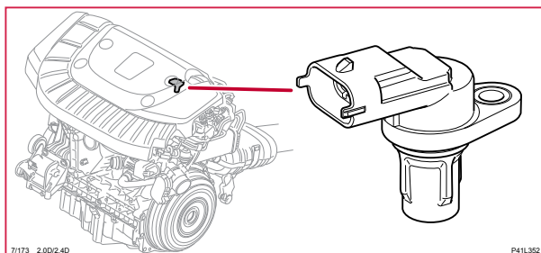
7/173 Lägesgivare kamaxel utloppssida, 5-CYL D
