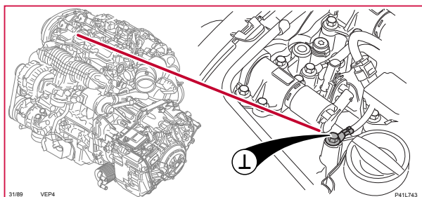
31/89 Stomanslutning, motor tändspolar, 4-CYL P
