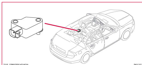
7/115 Sidokrockgivare vänster B-stolpe, S60
