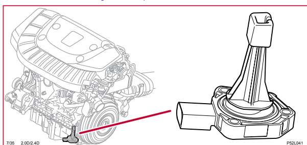
7/35 Givare oljenivå, 5-CYL D
