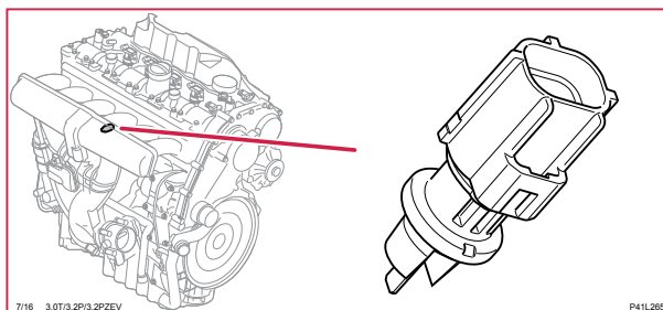
7/16 Givare kylvätsketemperatur, 6-CYL
