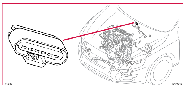
74/316 Kontaktstycke, BK, STOSTA
