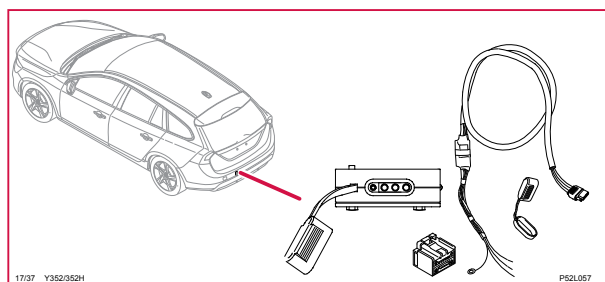
17/37 Uttag 4-poligt, ledningsmatta dragkrok, V60
