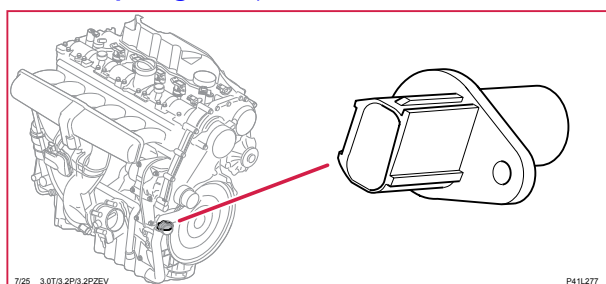
7/25 Impulsgivare, 6-CYL
