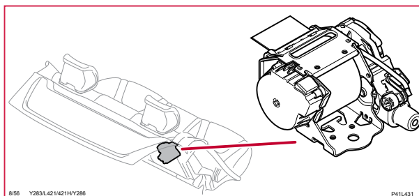
8/56 Tändare bältessträckare bak höger, S60
