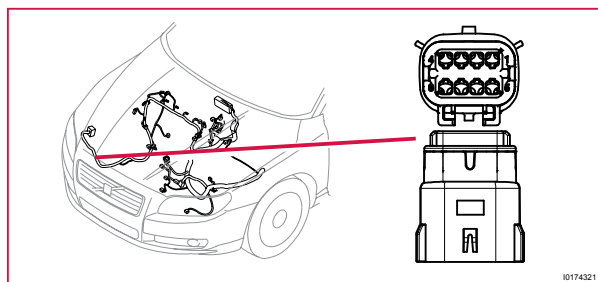
74/321 Kontaktstycke, BK
