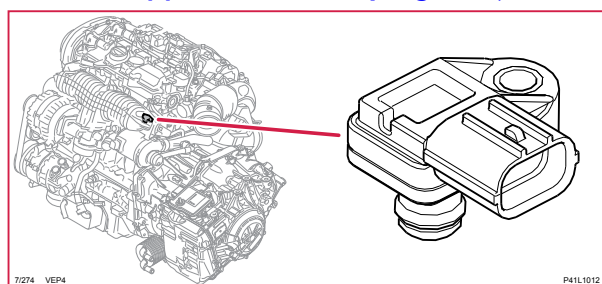
7/274 Inloppsrör absoluttryckgivare, 4-CYL P
