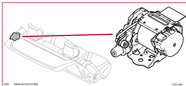
8/55 Tändare bältessträckare bak vänster, S60
