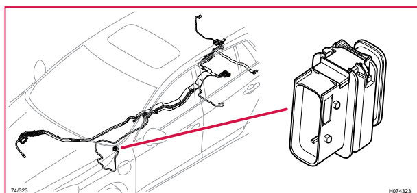
74/323 Kontaktstycke, BK
