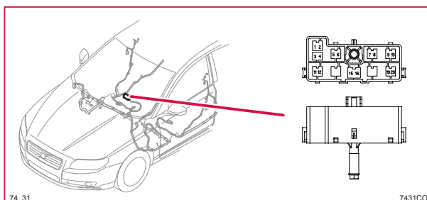
74/31 Kontaktstycke, BK
