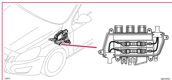
11P/1 Säkringar, laddanslutning
