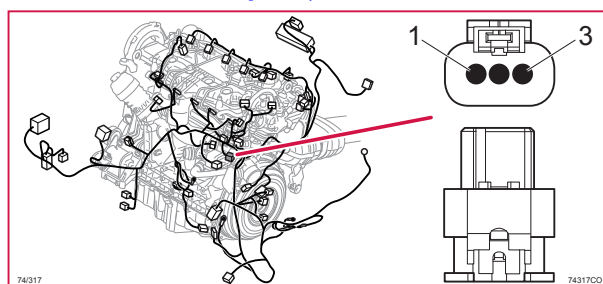
74/317 Kontaktstycke, BK
