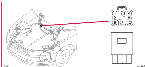
74/9 Kontaktstycke, BK
