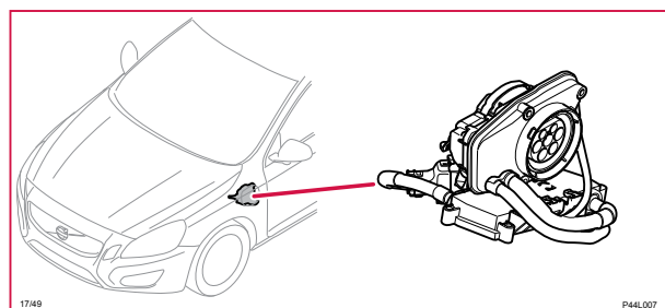
17/49 Laddningsanslutning
