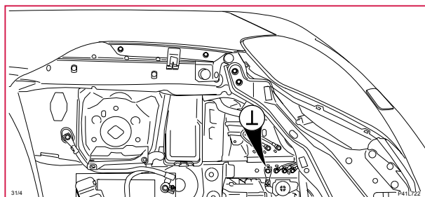
31/4 Stomanslutning, Motor
