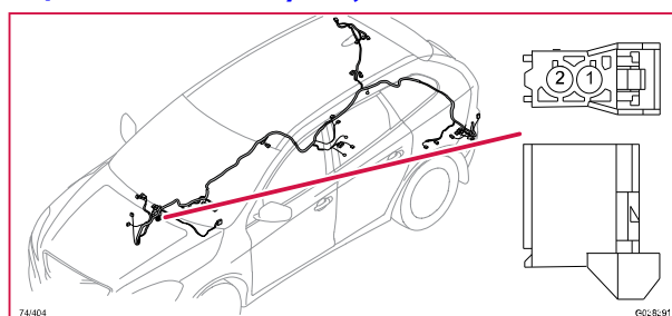
74/404 Kontaktstycke, BK
