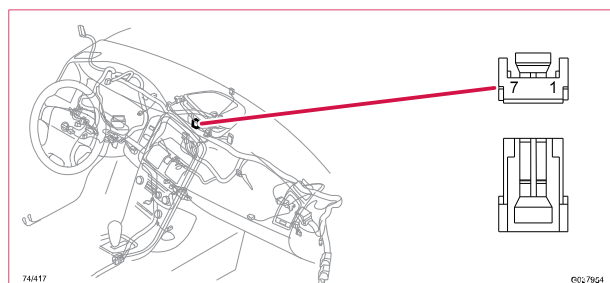
74/417 Kontaktstycke, GN, V60H
