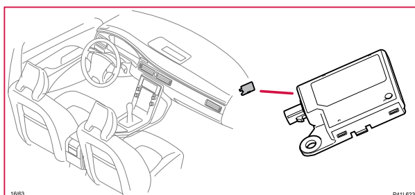
16/63 GPS-antenn mobiltelefon
