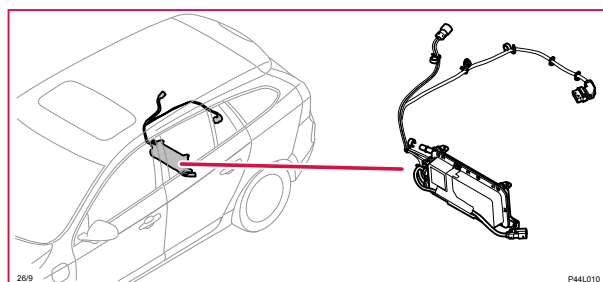
26/9 Batteriladdare (OBC)
