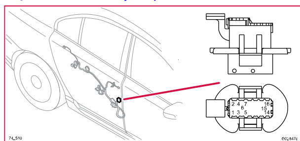
74/510 Kontaktstycke, BK
