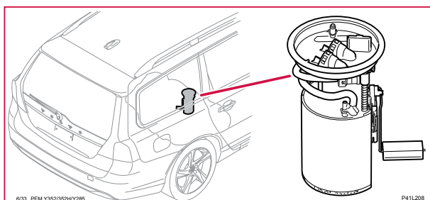
6/33 Bränslepump, V60H
