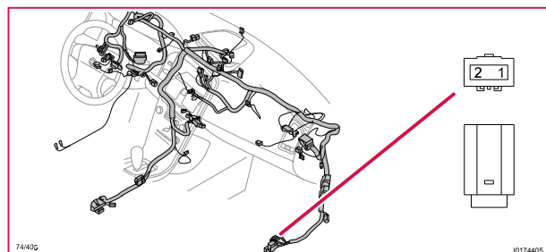
74/405 Kontaktstycke, WH
