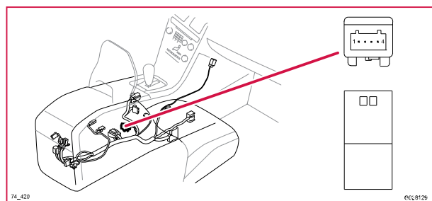
74/420 Kontaktstycke, GY
