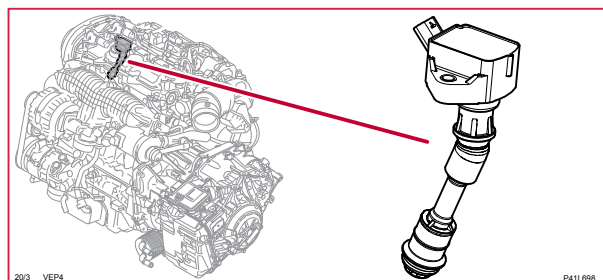
20/3-6 Tändstift med tändspolar, S60LH
