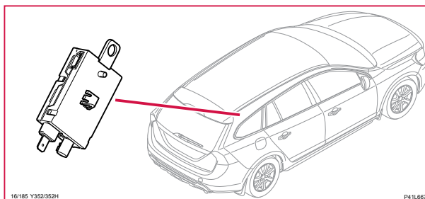
16/185 TV-Antenn, V60H
