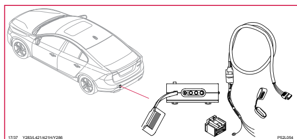
17/37 Uttag 4-poligt, ledningsmatta dragkrok, S80
