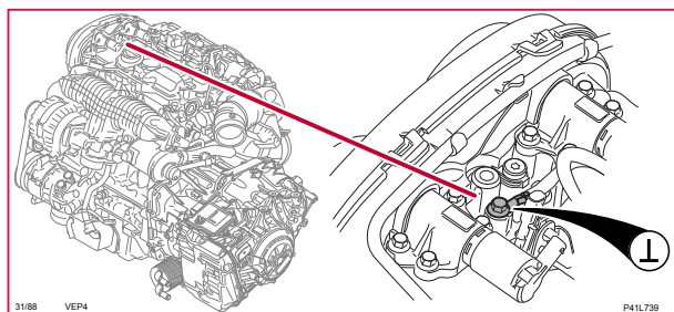
31/88 Stomanslutning, motor tändspolar, 4-CYL 2.0P
