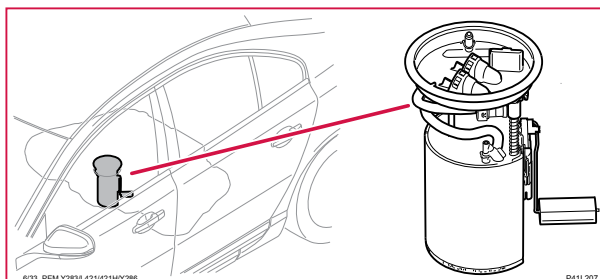
6/33 Bränslepump, S80
