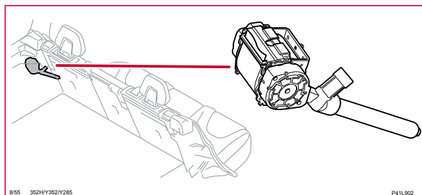
8/55 Tändare bältessträckare bak vänster, V70, XC70
