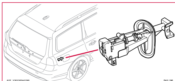
6/37 Låsmotor tanklucka, V70, XC70
