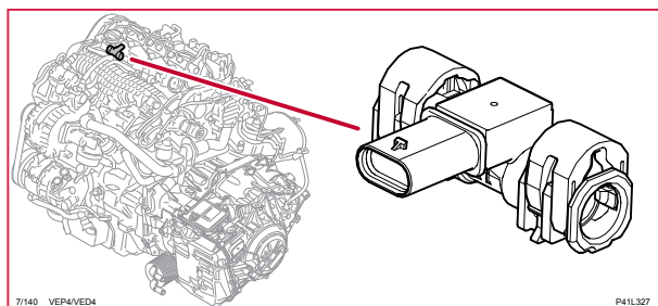
7/140 Bränsletryckgivare låg, 4-CYL 2.0L
