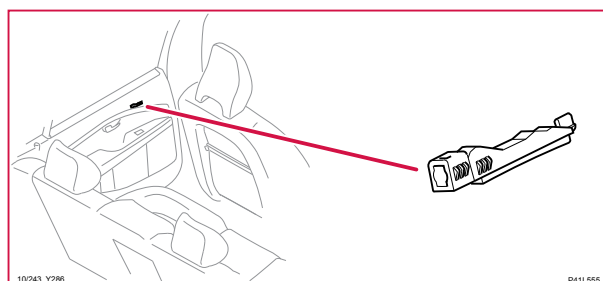
10/243 Lampa, inre dörrhandtag, bakre vänster
