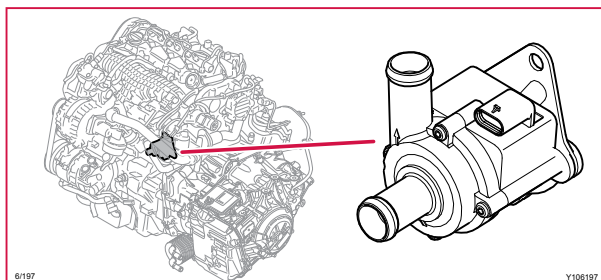
6/197 EGR-kylpump
