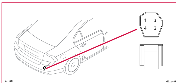
74/523 Kontaktstycke, GY, PDC
