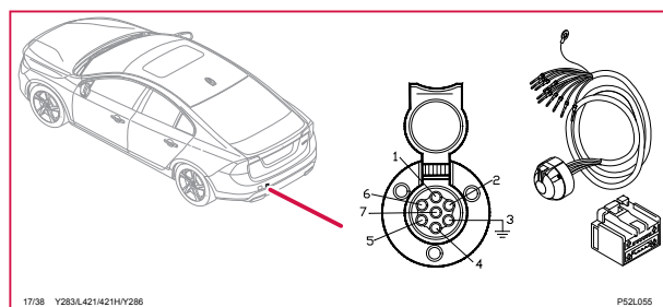
17/38 Uttag 7-poligt, ledningsmatta dragkrok, S80
