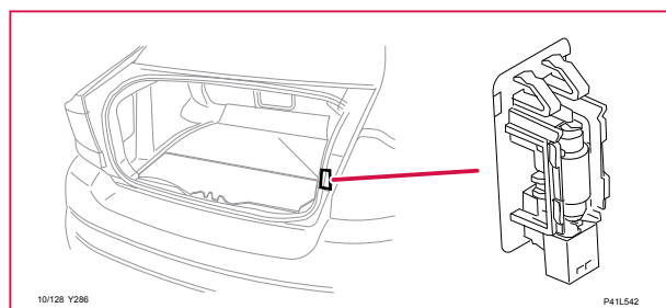
10/128 Lampa, bagageutrymme, höger, S80
