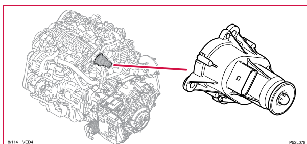
8/114 Virvelspjällventil, 4-CYL 2.0D
