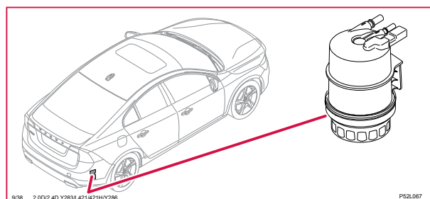
9/38 Eluppvärmt bränslefilter, S80
