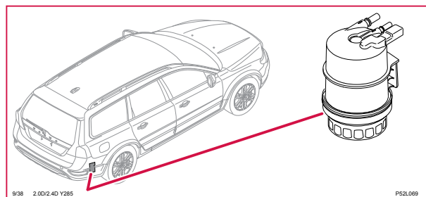
9/38 Eluppvärmt bränslefilter, V70, XC70
