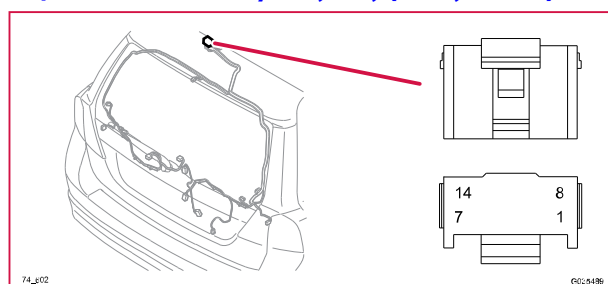
74/602 Kontaktstykke, GY, (V70, XC70)
