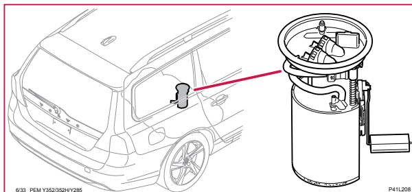
6/33 Bränslepump, V70, XC70
