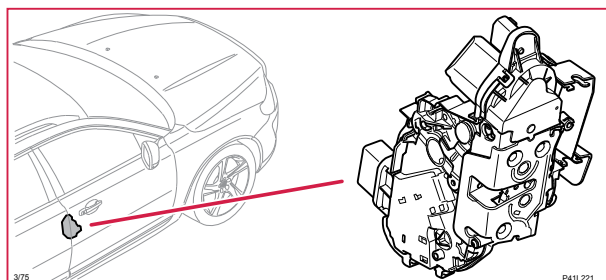
3/75 Låsenhet, höger framdörr
