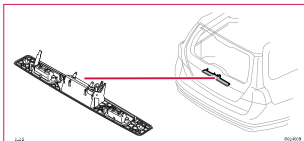
3/35 Omkopplare, bagageutrymmets handtag, V70, XC70
