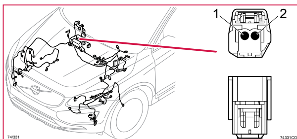
74/331 Kontaktstycke, BK
