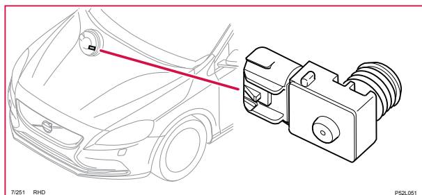
7/251 Bromsvakuumgivare, RHD
