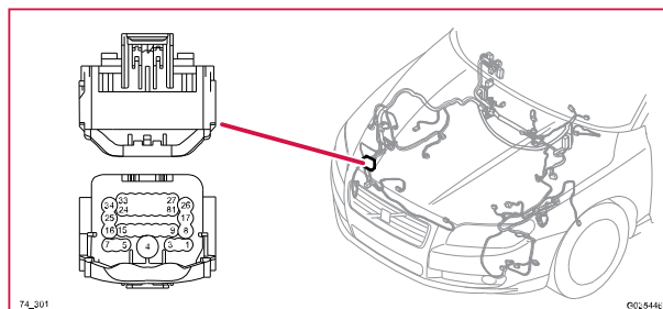
74/301 Kontaktstycke, BK
