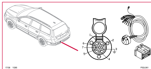
17/38 Uttag 7-poligt, ledningsmatta dragkrok, V70, XC70
