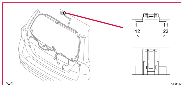
74/603 Kontaktstykke, GY, (V70, XC70)
