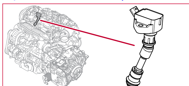
20/3-8 Tändstift med tändspolar
