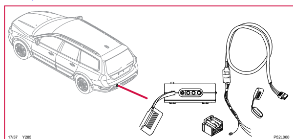
17/37 Uttag 4-poligt, ledningsmatta dragkrok, V70, XC70
