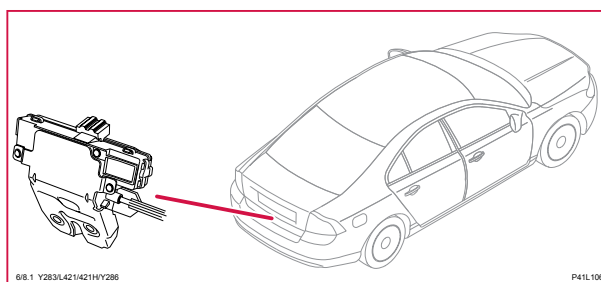
6/8 Centrallåsmotor, bagageutrymme, S80
