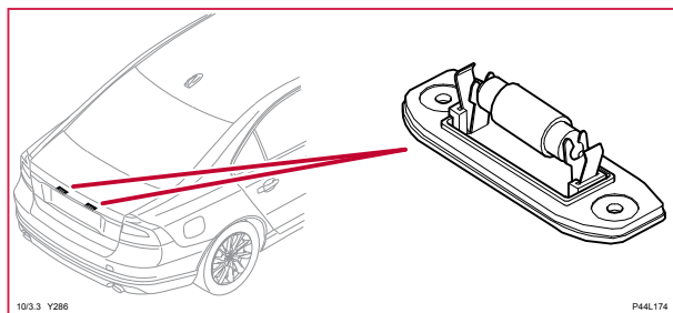
10/3 Skyltbelysning, S80
