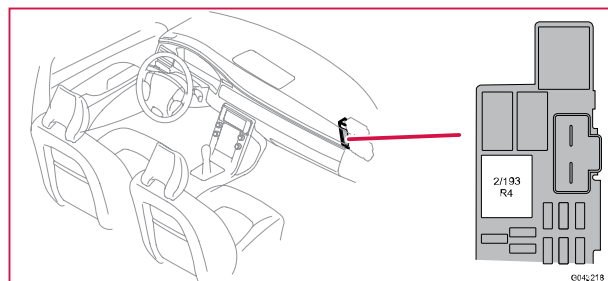
2/246 Relä, sekundärbatteri
