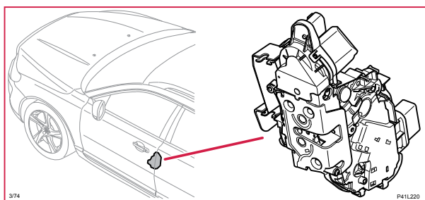
3/74 Låsenhet, vänster framdörr
