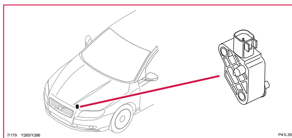
7/179 Frontkrockgivare vänster
