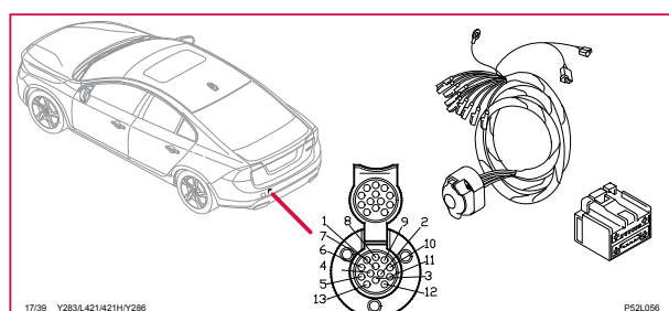
17/39 Uttag 13-poligt, ledningsmatta dragkrok, S80
