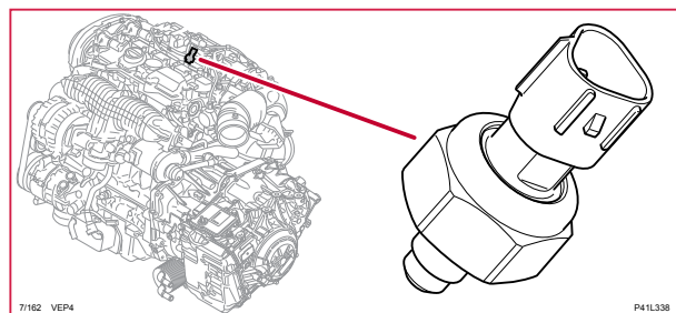
7/162 Tryckgivare bränslerör, 4-CYL 2.0P
