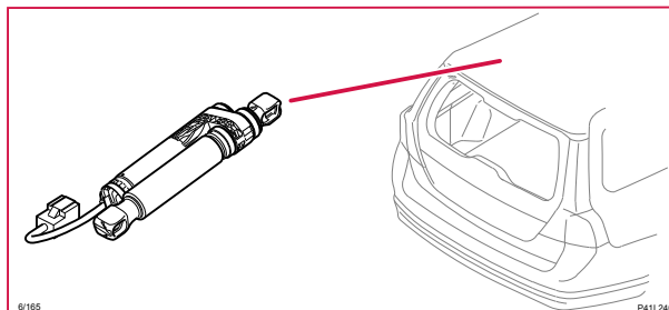
6/165 Motor, bakluckeöppning, vänster
