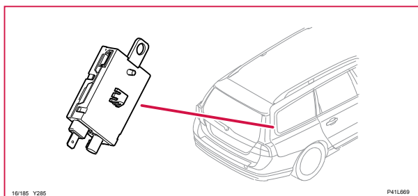
16/185 TV-Antenn, V70, XC70
