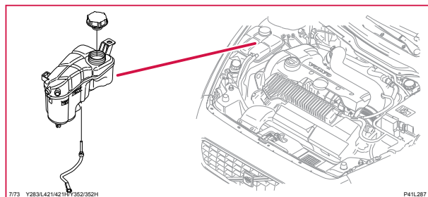
7/73 Givare, kylvätskenivå
