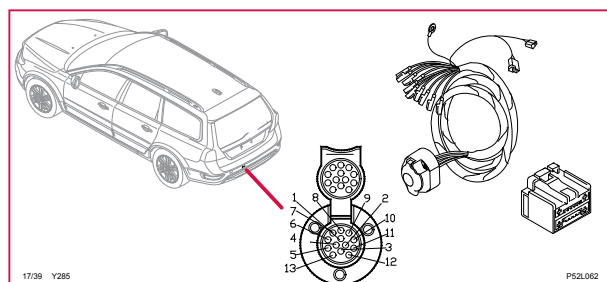
17/39 Uttag 13-poligt, ledningsmatta dragkrok, V70, XC70
