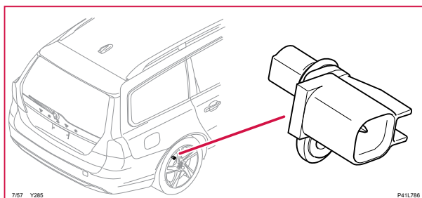
7/57 Givare, ABS, bakre höger, V70, XC70
