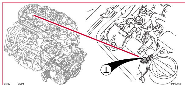
31/89 Stomanslutning, motor tändspolar, 4-CYL 2.0P
