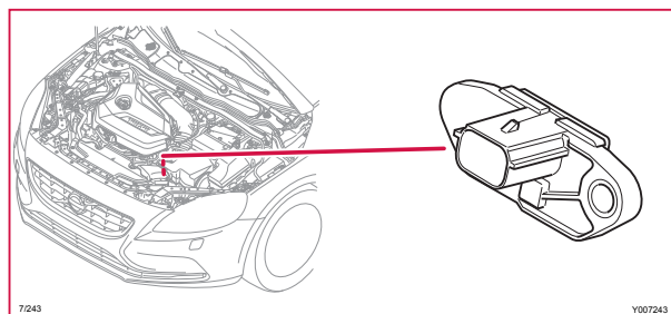
7/243 Växlgivare neutralläge, 4-CYL 2.0D
