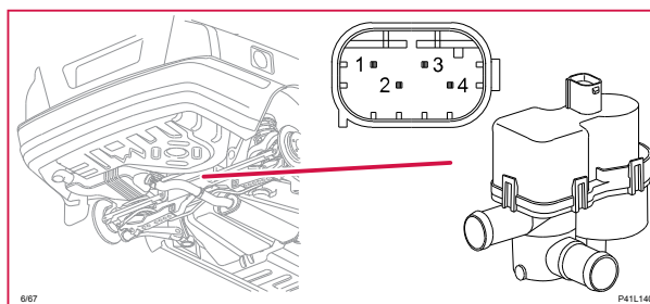
6/67 Pump bränsleläckagekontroll
