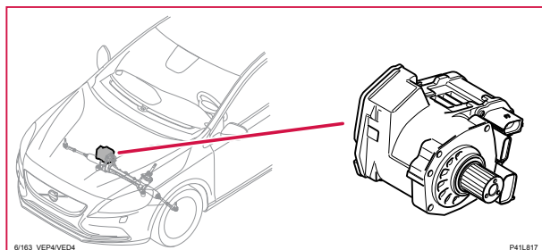
6/163 Elektrisk styrservoehet (PSCM), EPAS
