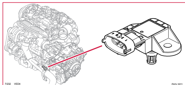
7/232 Inloppsörsluft temperatur- och tryckgivare, 4-CYL 2.0D
