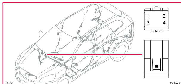
74/534 Kontaktstykke, GY, AUD
