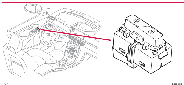
3/81 Omkopplare, elektriska fönsterhissar, förardörr
