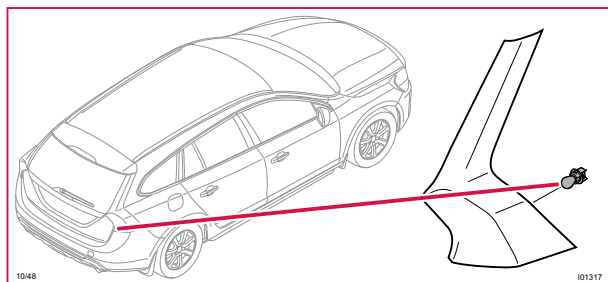
10/48 Backljus höger
