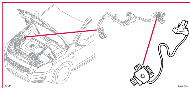
8/185 Klimatavstängningsventil
