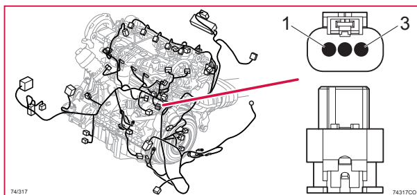
74/317 Kontaktstycke, BK
