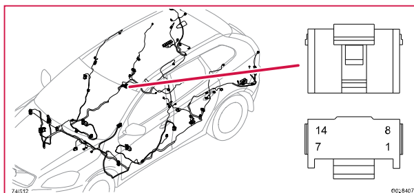
74/512 Kontaktstycke, GY
