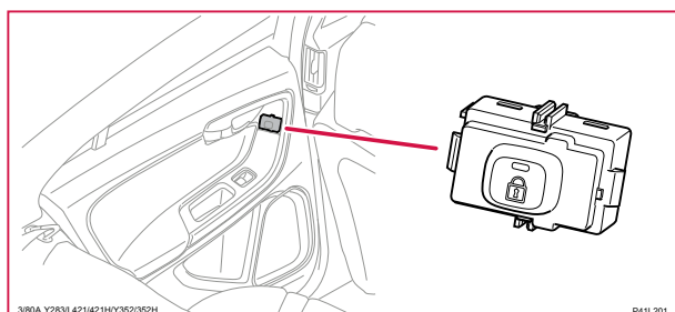
3/80A Omkopplare, centrallåssystem, vänster bakdörr
