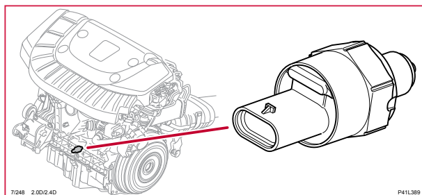
7/248 Oljetryck och temperaturgivare
