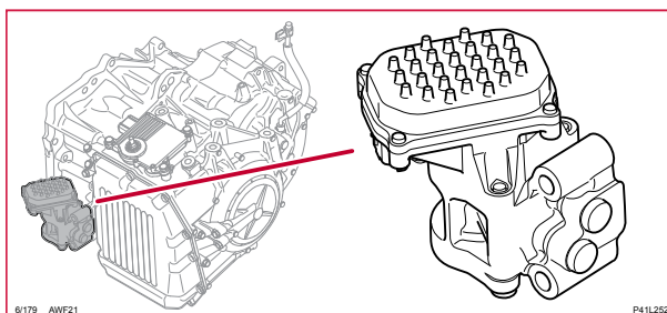
6/179 Elektrisk oljepump
