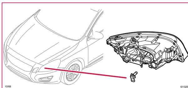
10/68 Hellsjus vänster
