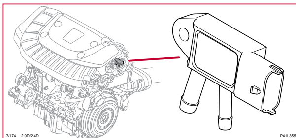
7/174 Tryckgivare, partikelfilter
