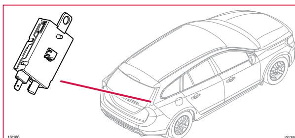
16/186 TV-Antenn
