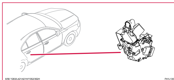
6/56 Motor, centrallås, höger baddörr
