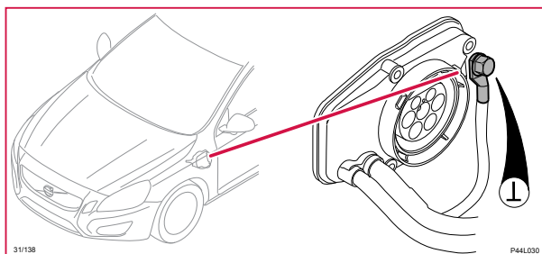
31/138 Skyddsjord laddanslutning
