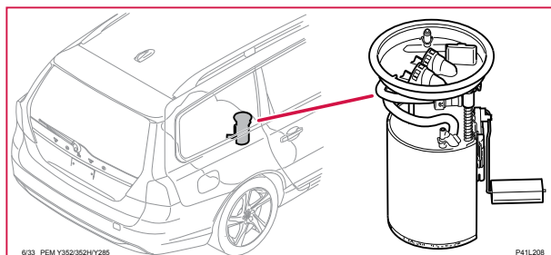
6/33 Bränslepump
