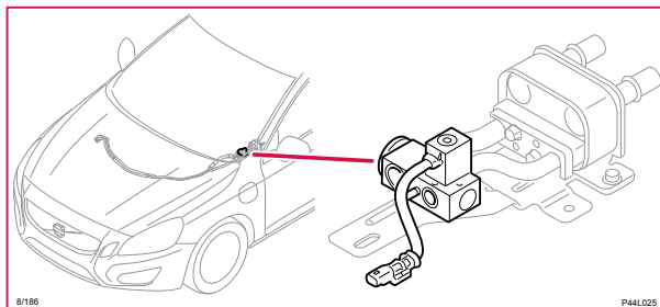
8/186 Avstängningsventil kylmedium
