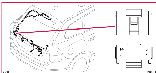
74/602 Kontaktstycke, GY
