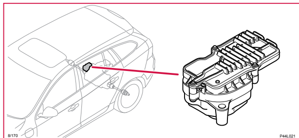
8/170 ERAD-koppling
