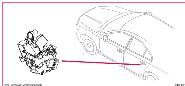
6/57 Motor, centrallås, baddörr vänster
