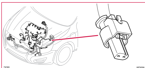
74/324 Kontaktstycke, BK
