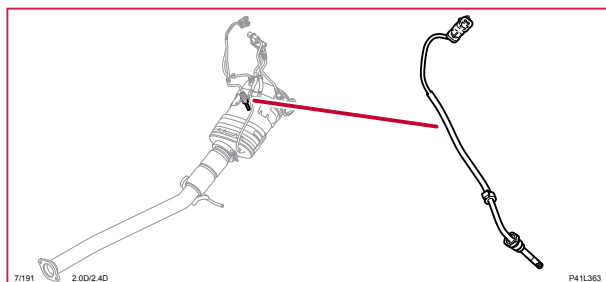
7/191 Temperaturgivare partikelfilter
