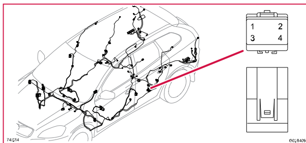
74/514 Kontaktstycke, GY
