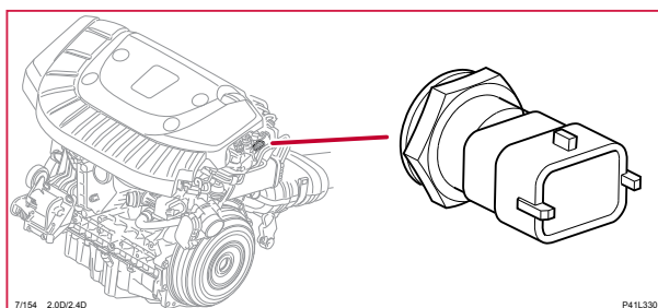
7/154 Givare bränsletemperatur
