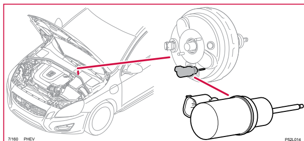
7/160 Bromsvakuumgivare
