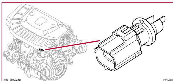
7/16 Givare kylväsketemperatur
