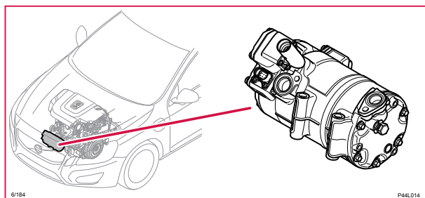
6/184 Elektrisk AC-kompressor
