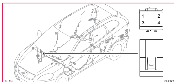
74/534 Kontaktstycke, GY, AUD
