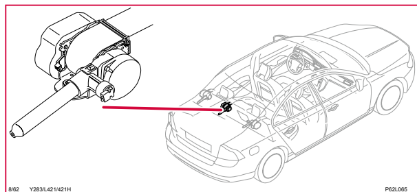
8/62 Tändare, bältessträckare, mittre baksäte
