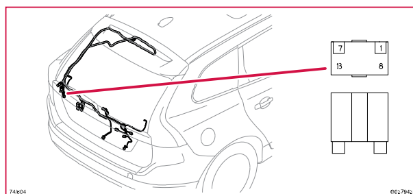
74/604 Kontaktstycke, GY
