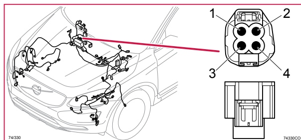
74/330 Kontaktstycke, BK
