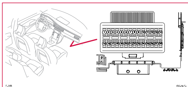
F/no. Säkringar
