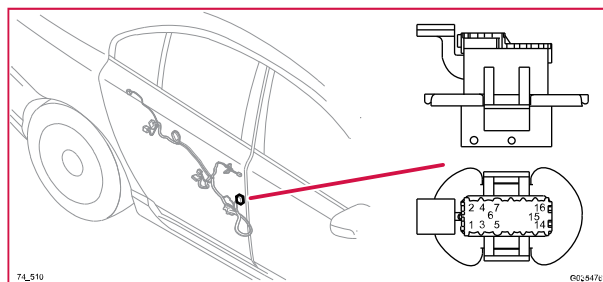
74/510 Kontaktstykke, BK
