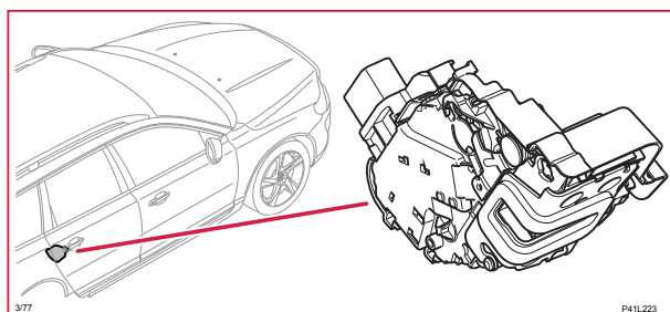
3/77 Låsenhet baddörr höger
