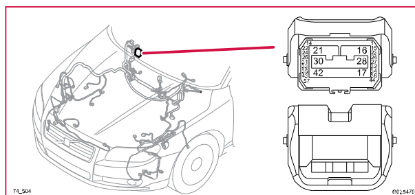
74/504 Kontaktstycke, NL
