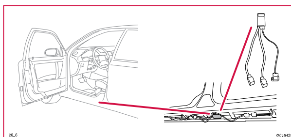
26/6 Omvandlare/styrenhet, instegslister, förarsida
