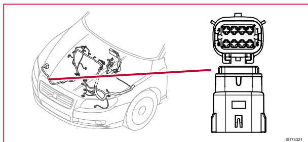
74/321 Kontaktstycke, BK
