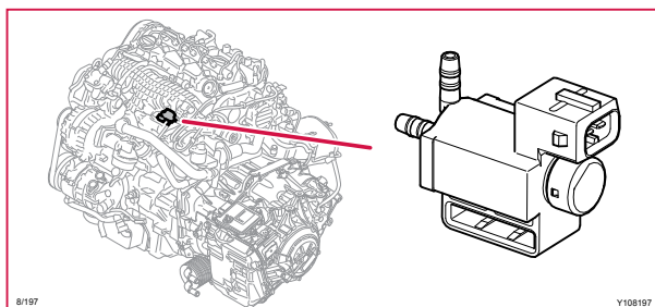
8/197 Vakuumpventil, vattenkyllar-bypass
