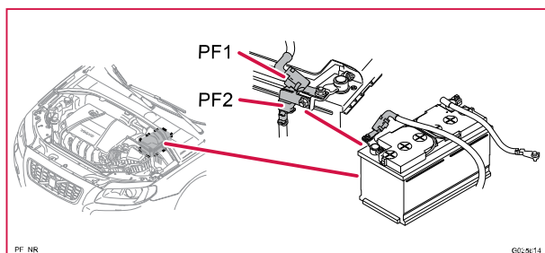
PF/no. Huvudsäkring vid batteri
