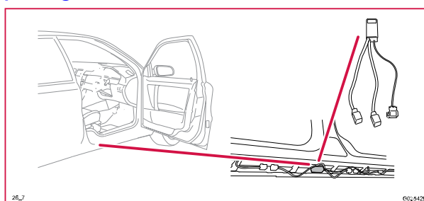
26/7 Omvandlare/styrenhet instegslister passagerarsida
