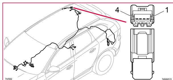
74/562 Kontaktstycke, BK
