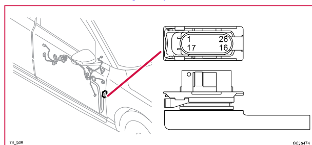
74/508 Kontaktstykke, BK
