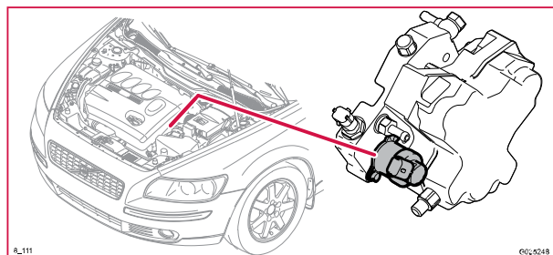
8/111 Reglerventil, bränsleflöde
