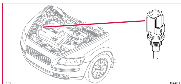
7/16 Givare kylväsketemperatur
