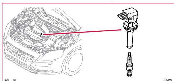
20/3-8 Tändstift med tändspolar
