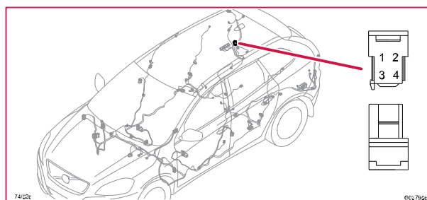
74/526 Kontaktstycke, GY
