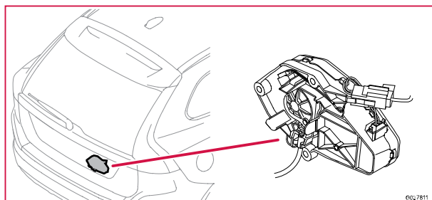
6/149 Motor stängning baklucka
