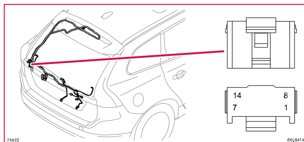
74/602 Kontaktstycke, GY
