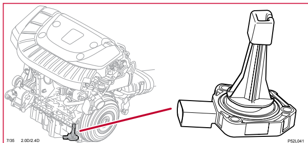
7/35 Givare oljenivå
