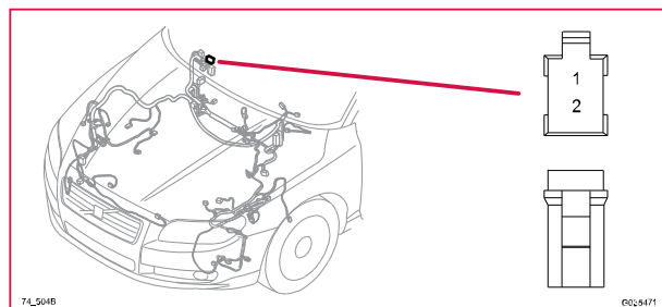
74/504B Kontaktstykke, RD
