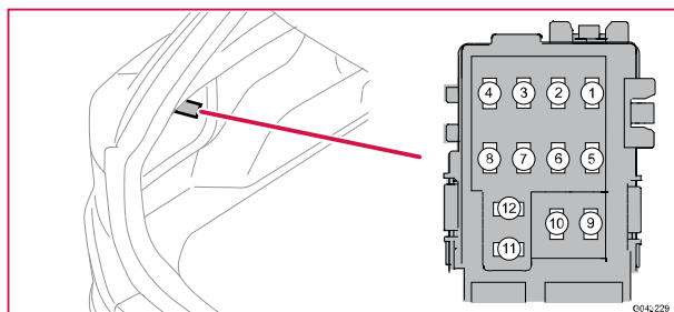
11D/A Säkringar, elcentral bagageutrymme A
