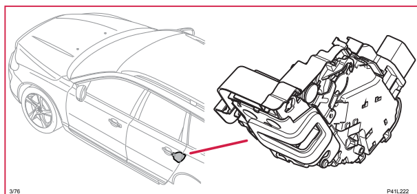
3/76 Låsenhet baddörr vänster
