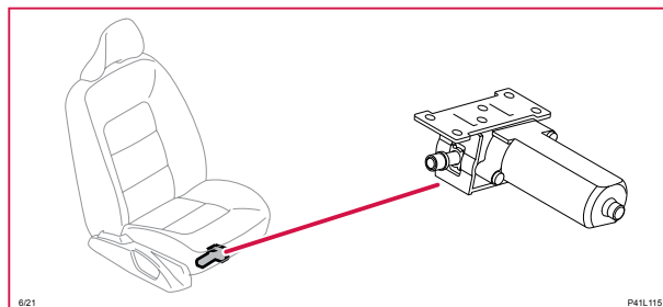
6/21 Sätsslutningsmotor, passagerarsida
