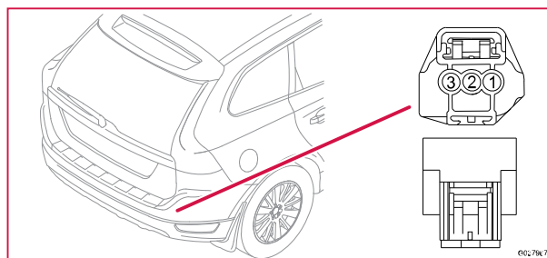
74/527 Kontaktstycke, BK
