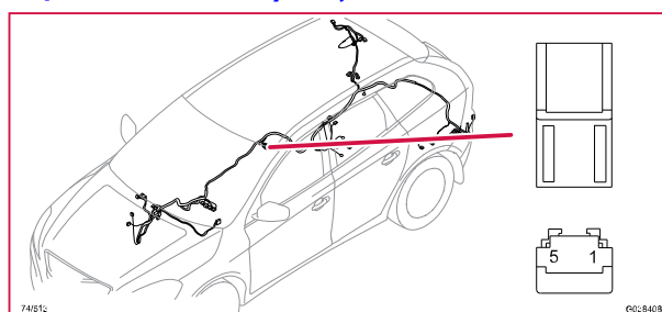
74/513 Kontaktstykke, GN
