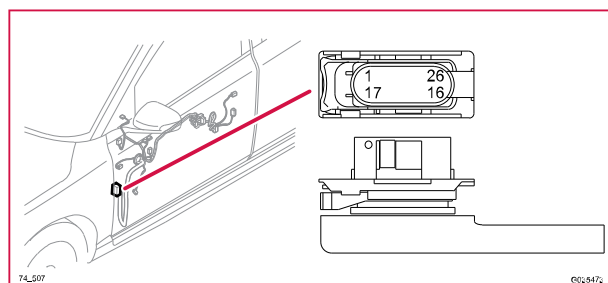
74/507 Kontaktstykke, BK
