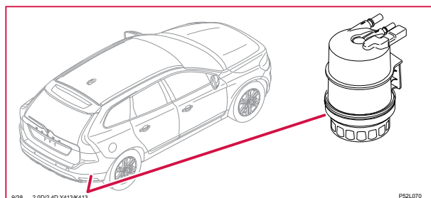
9/38 Eluppvärmt bränslefilter
