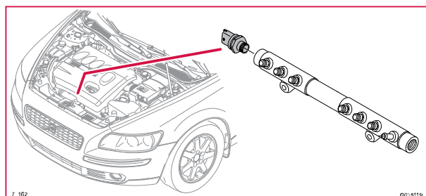
7/162 Tryckgivare bränslerör
