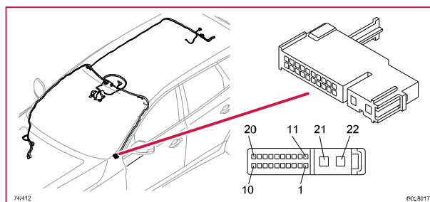
74/412 Kontaktstycke, GN
