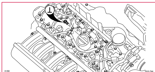
31/90 Stomanslutning, motor tändspolar, 6-CYL
