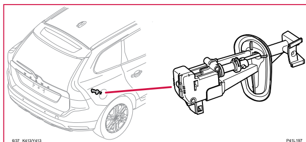
6/37 Låsmotor tanklucka
