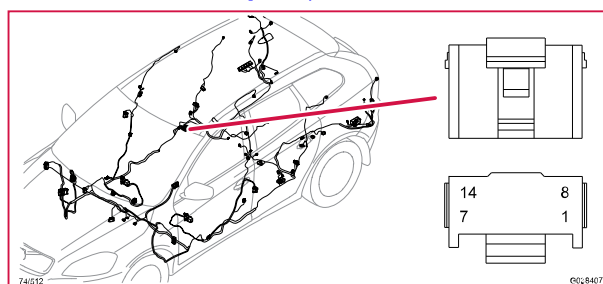
74/512 Kontaktstykke, GY
