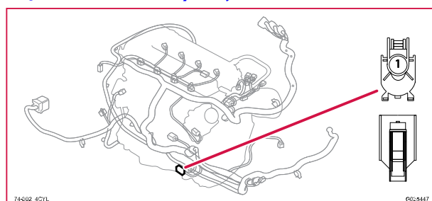
74/302 Kontaktstycke, BK
