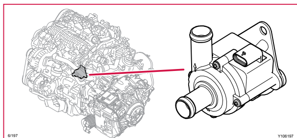
6/197 EGR-kylpump
