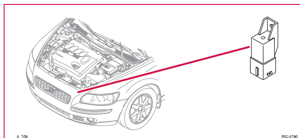
4/109 Styrenhet glödstift
