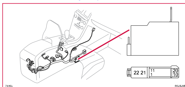
74/503 Kontaktstycke, GY
