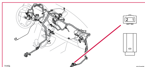
74/405 Kontaktstycke, BK
