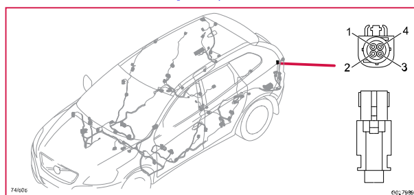
74/606 Kontaktstycke, BK
