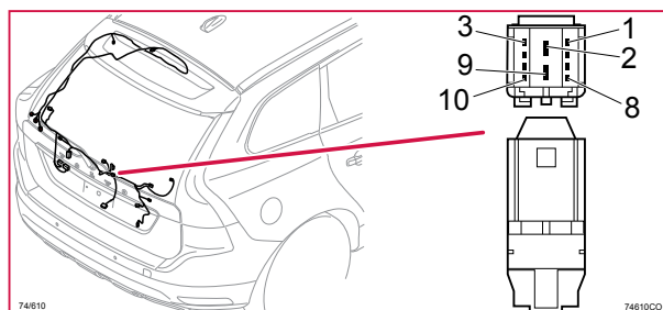
74/610 Kontaktstycke, GY
