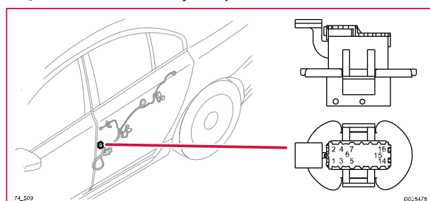
74/509 Kontaktstykke, BK
