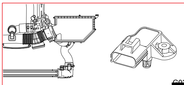
7/165 Tryck- och temperaturgivare inloppsrör, DIESEL
