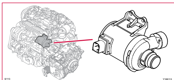
6/113 Kylvattenpump
