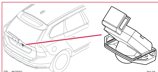
27/6 Kamera
