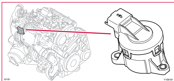
6/181 Laddluftkompressor-bypass ställdon
