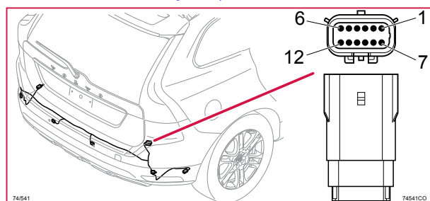
74/541 Kontaktstycke, BK
